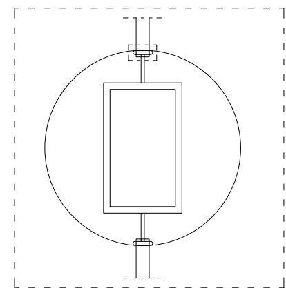
DETALLE SUJECIÓN BOLA PVC A BARRA METALICA
