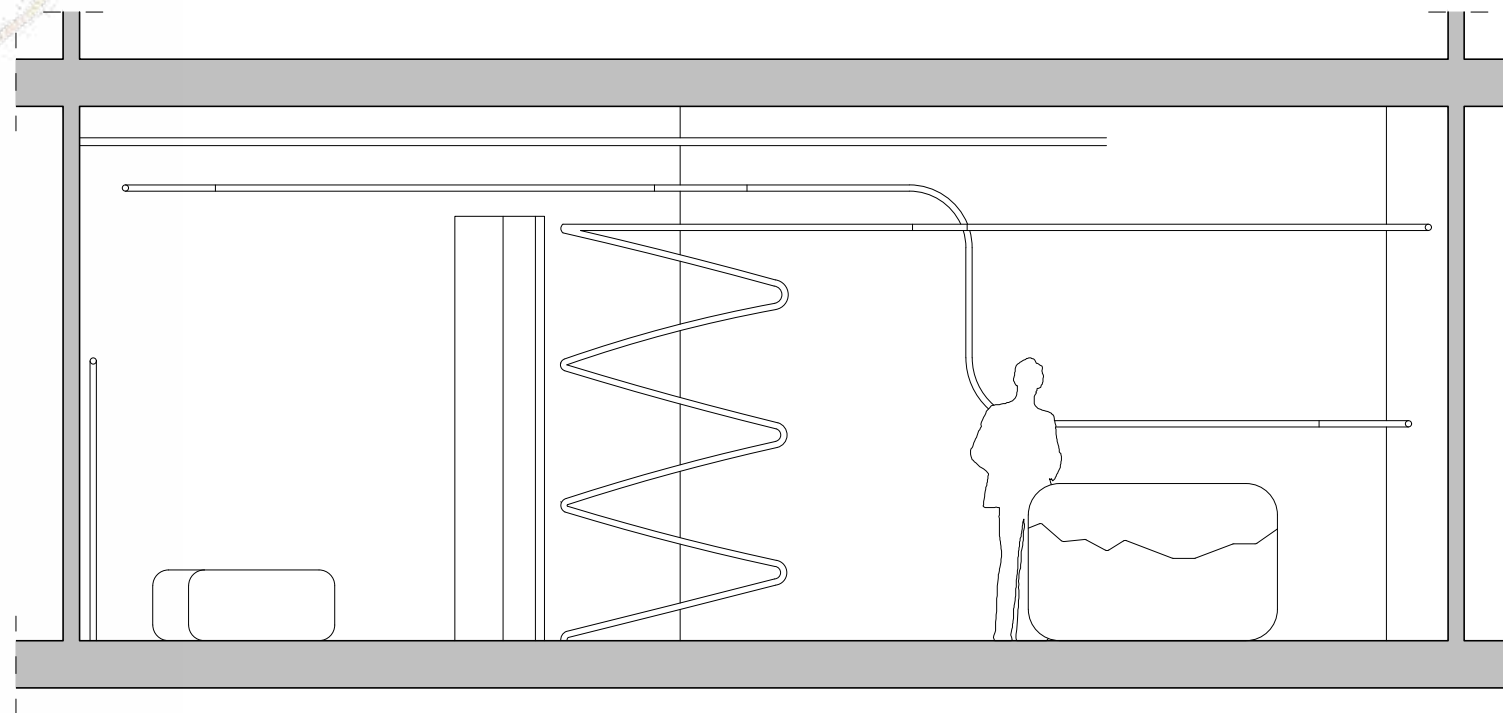
SECCIÓN AA'
