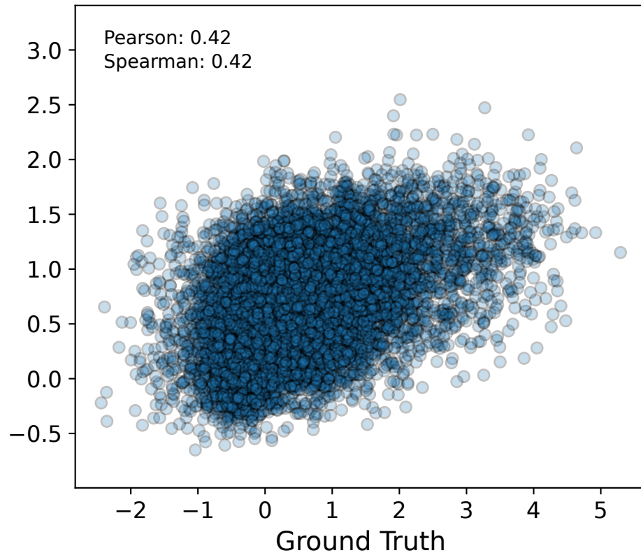
model_500
