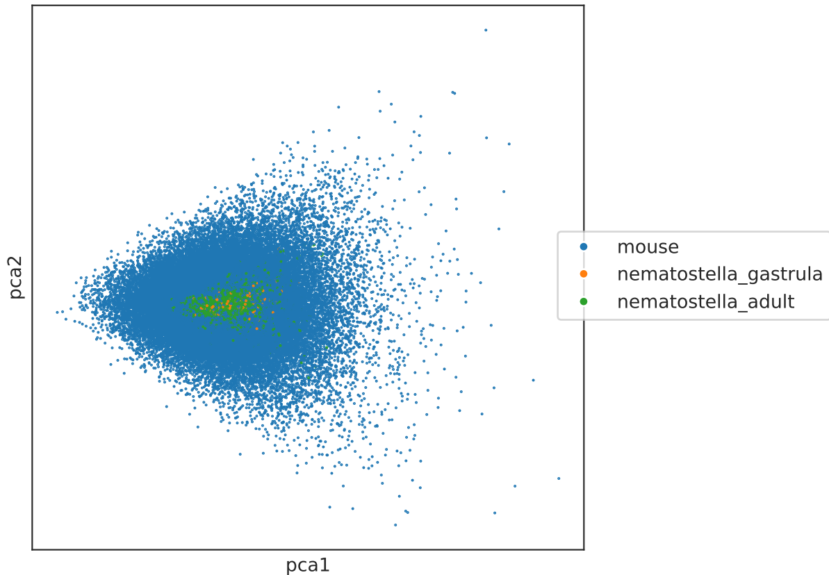
PCA Species (centered-sum)
