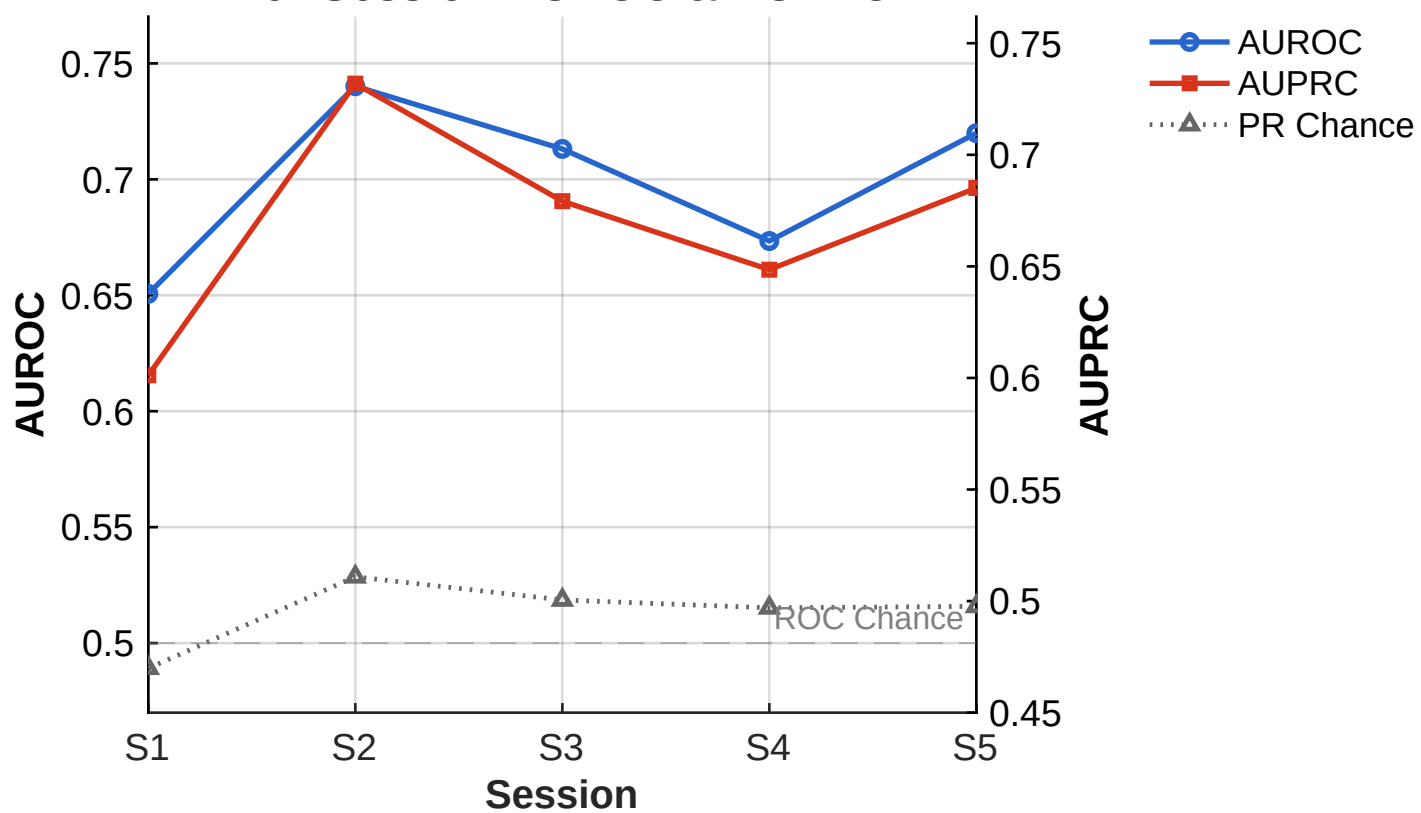
Per-Session AUROC & AUPRC
