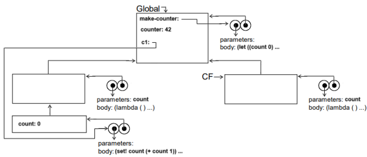
Step10 (let ((count 0) ...) ...)
