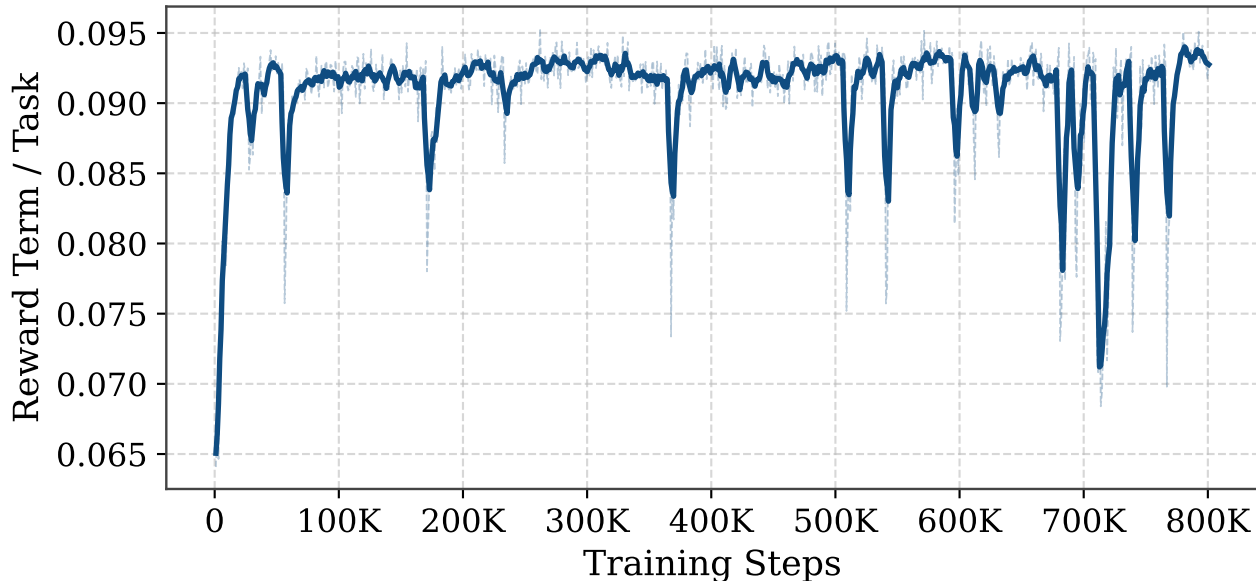
QoS Reward per Task
