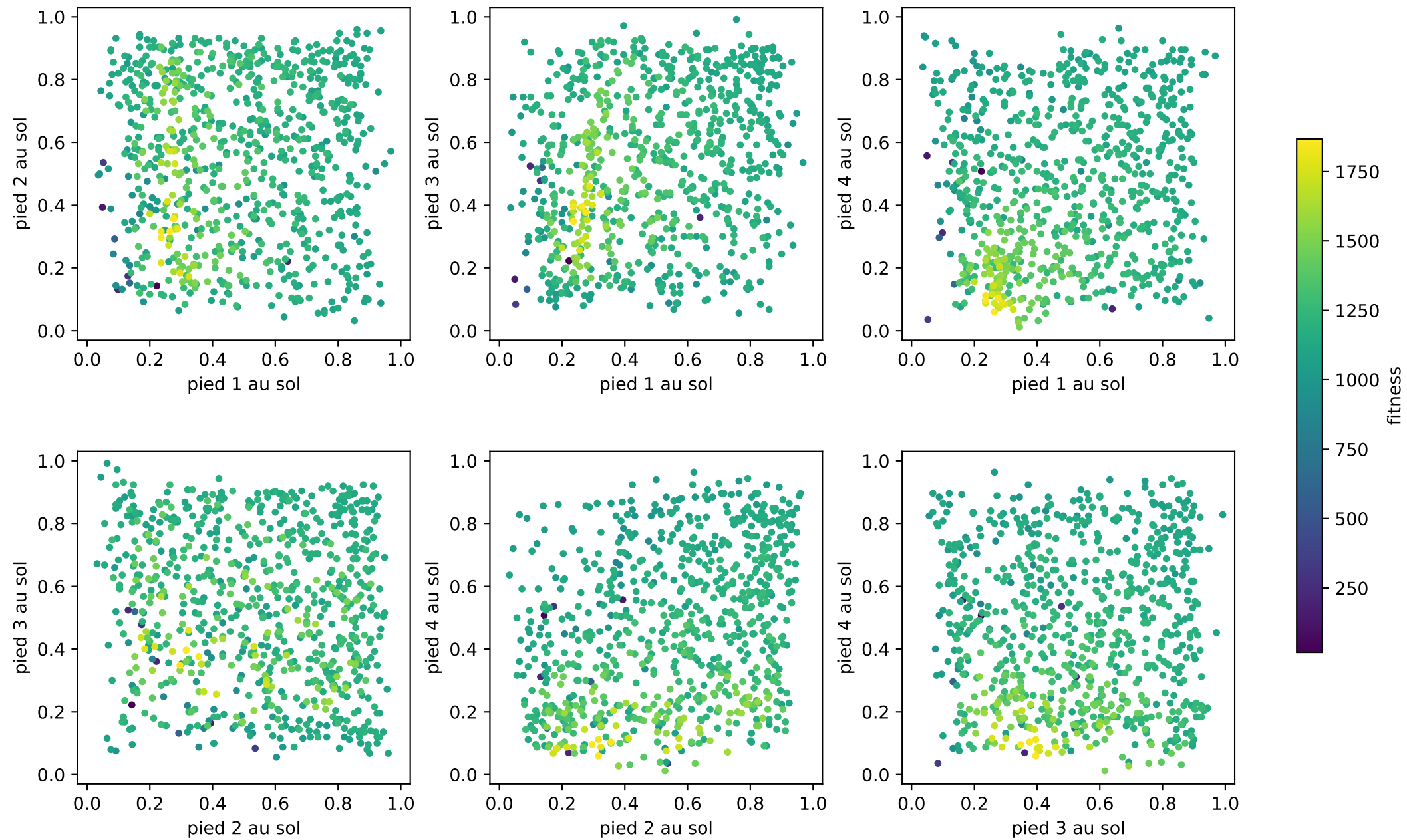
PGA-ME (seed 0) — 786 démarches dans le répertoire
