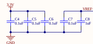
STM32电源部分 STM32 Power supply
