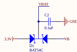
RTC电源 RTC circuit
