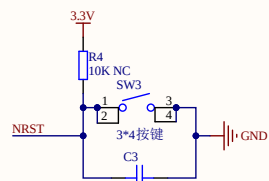
复位电路 Reset circuit
