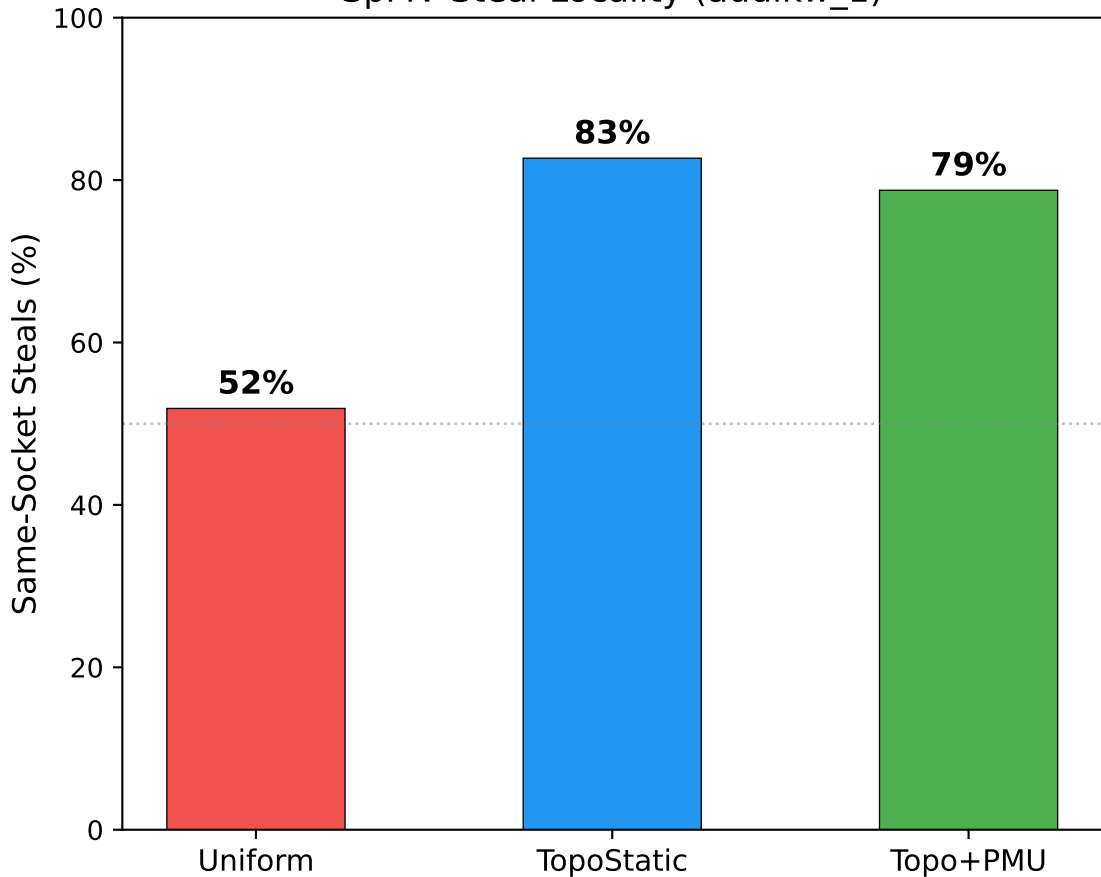
SpMV Steal Locality (audikw_1)
