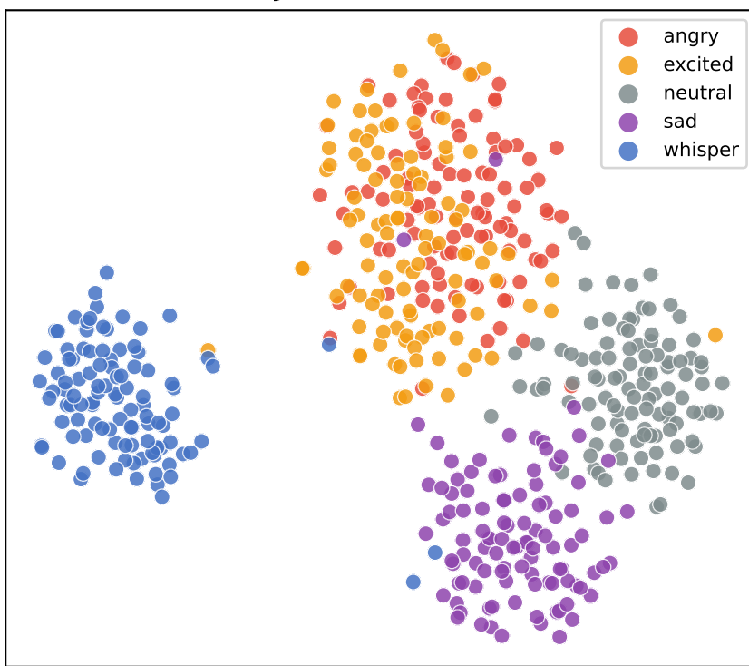
JEPA-EMA (v9)
