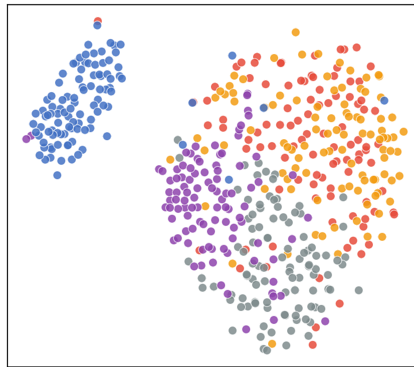
EnCodec
