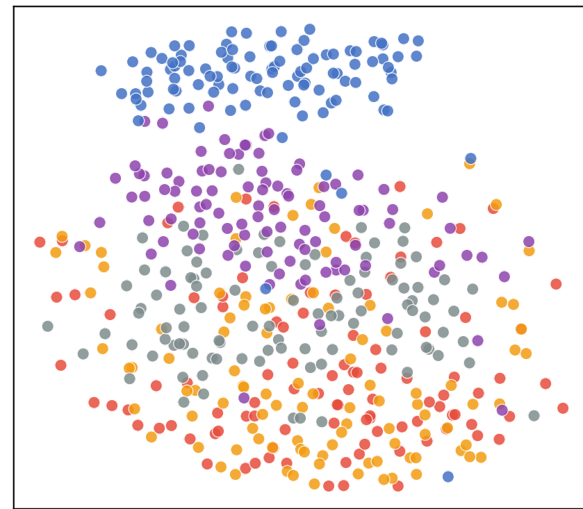
DAC
