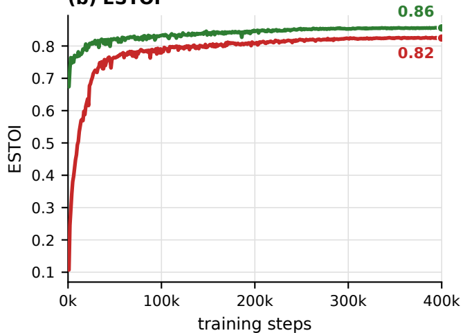
(b) ESTOI
