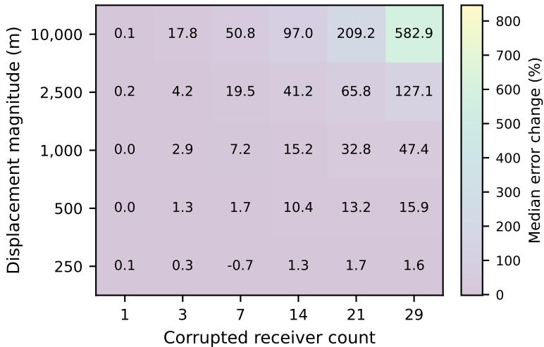
(d) Min-Max
