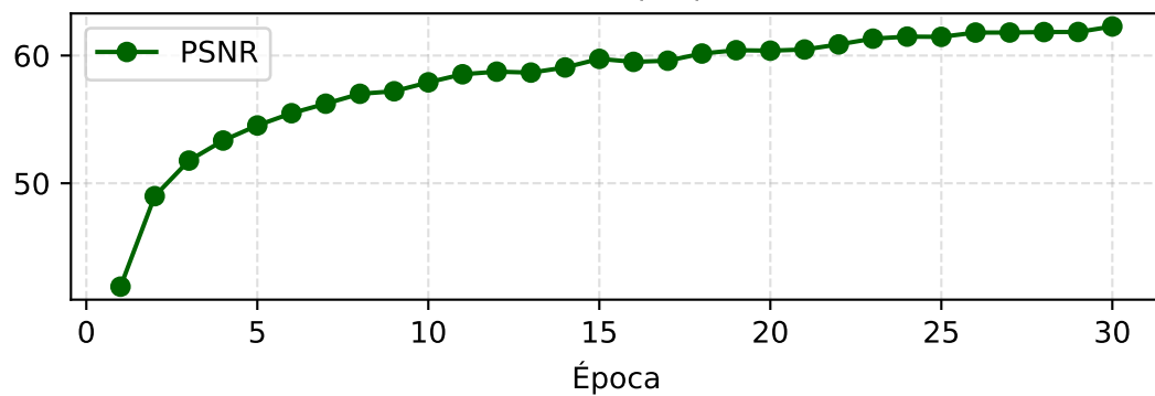
PSNR (dB)
