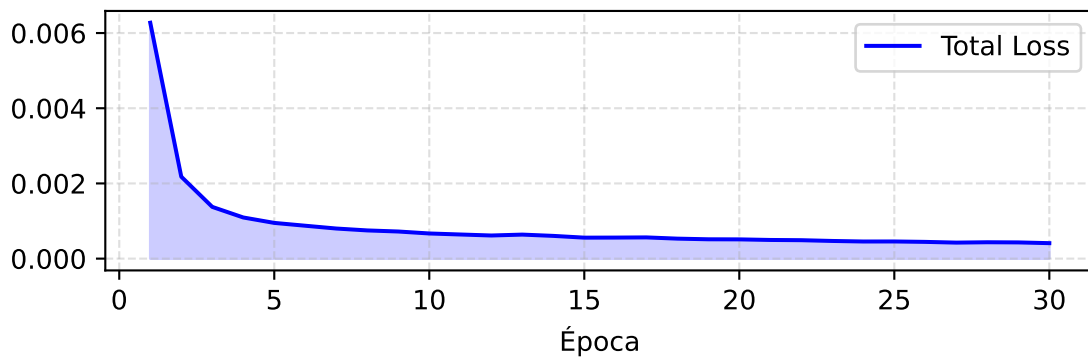
L1 (MAE)
