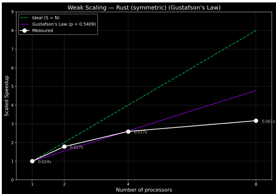
Слика 11: Скалирано убрзање при слабом скалирању — симетрично стабло, Rust
