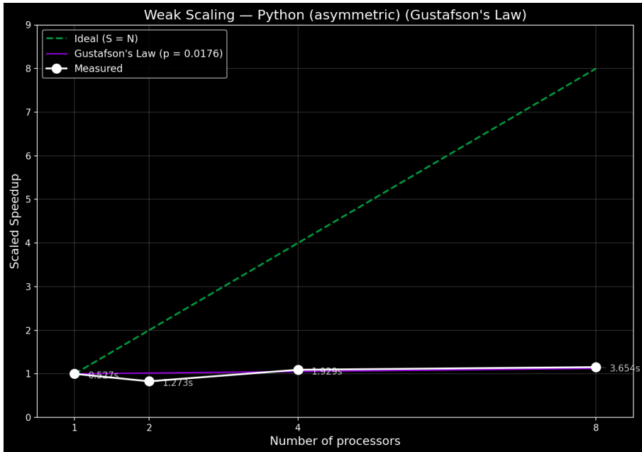
Слика 12: Скалирано убрзање при слабом скалирању — асиметрично стабло, Python
