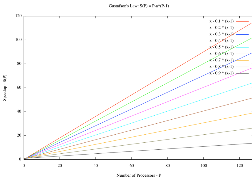
Слика 5: Амдалов закон (горе) — убрзање асимптотски тежи 1/f [17]; Густафсонов закон (доле) — убрзање расте линеарно са бројем процесора [18].
