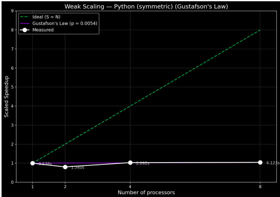
Слика 10: Скалирано убрзање при слабом скалирању — симетрично стабло, Python
