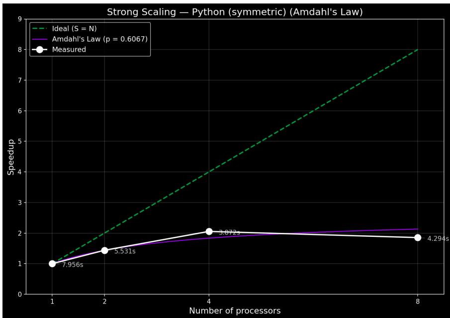
Слика 6: Убрзање при јаком скалирању — симетрично стабло, Python
