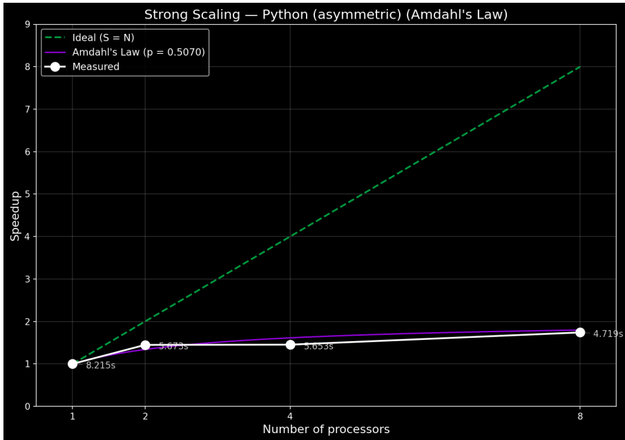
Слика 8: Убрзање при јаком скалирању — асиметрично стабло, Python
