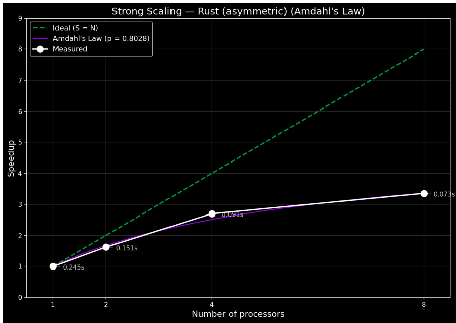
Слика 9: Убрзање при јаком скалирању — асиметрично стабло, Rust
