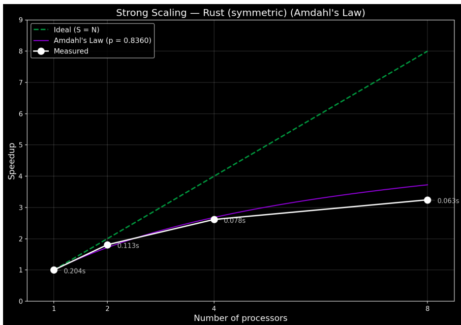
Слика 7: Убрзање при јаким скалирању — симетрично стабло, Rust
