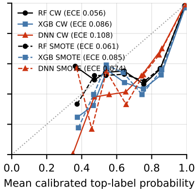
UNSW-NB15
