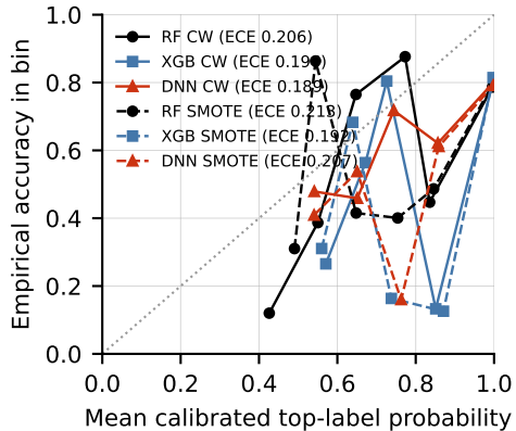
NSL-KDD
