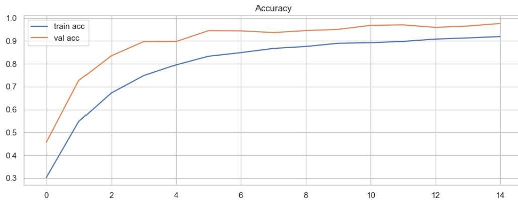
Fig. 3. – Courbe d'accuracy du CNN sur GTSRB (entraînement vs validation).
