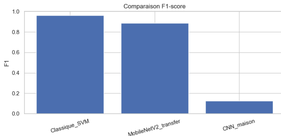
Fig. 7. – Comparaison des scores F1 sur le dataset local.
