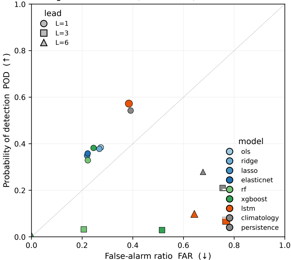
Categorical extremes (truth &lt; -1.0) · LSTM vs default
