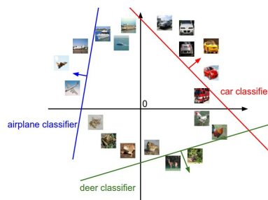
Linear classifier
