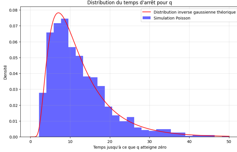
Figure 4 – Histogramme des temps d’arrêt simulés et densité IG théorique. Le test de Kolmogorov-Smirnov ne rejette pas l’hypothèse d’adéquation.
