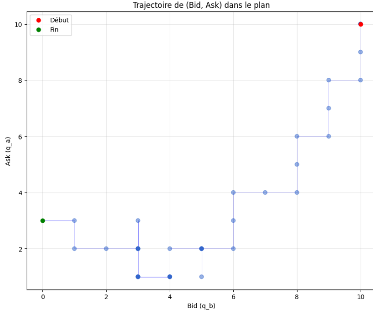
Figure 2 – Trajectoire dans le plan (q_b, q_a) jusqu'à ce qu'un côté atteigne zéro. Le point rouge marque le départ, le point vert l'arrêt.
