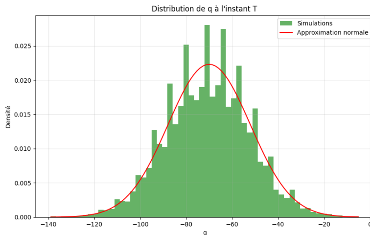
Figure 3 – Distribution empirique de q(T) contre \mathcal{N}(-70, 320) . Sans absorption, la marche aléatoire entière est très bien approchée par sa limite brownienne dès T = 100 .
