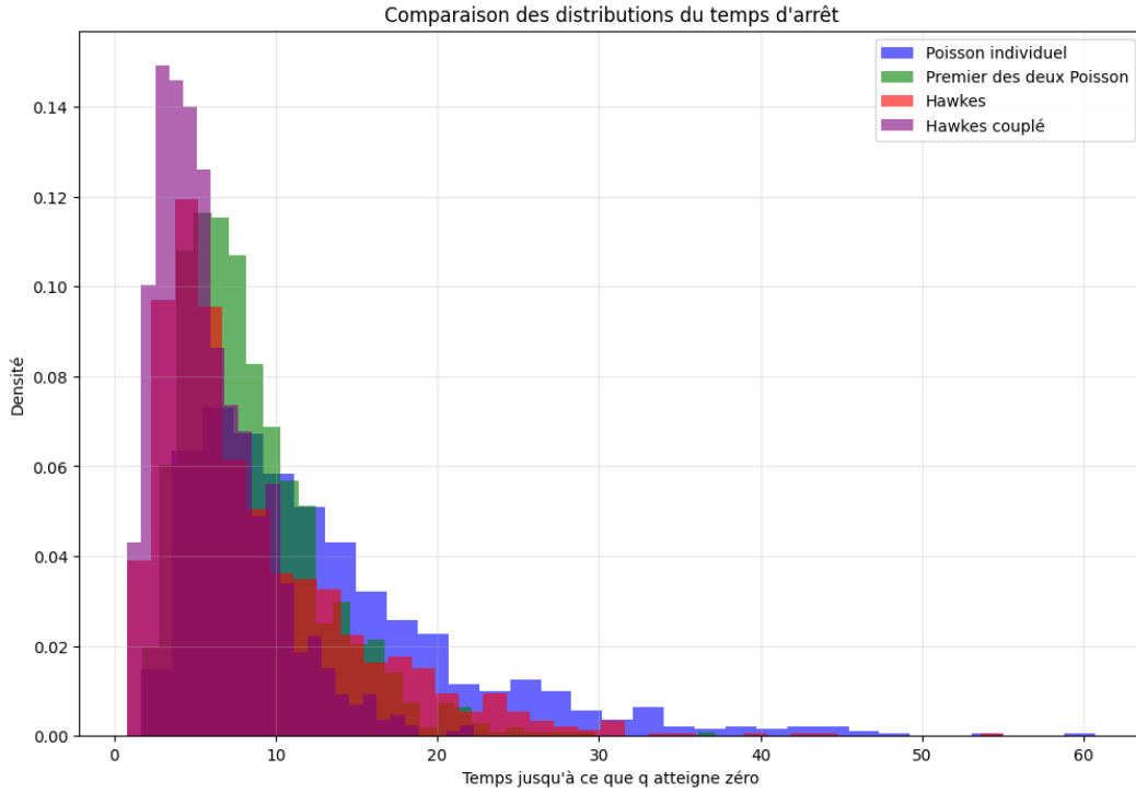
Figure 12 – Densités empiriques du temps d'arrêt pour les quatre régimes.
