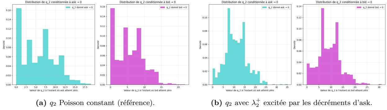
Figure 14 – Distribution conditionnelle de q_2(\tau) dans le cas symétrique ( \mu_a^- = \mu_b^- = 2 ). À gauche, modèle indépendant ; à droite, modèle couplé via les décréments d'ask.
