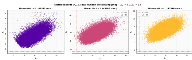
(a) États (\lambda_a^-, \lambda_b^-) aux niveaux k = 8, 5, 1 — côté bid. Les survivants ont \lambda_b^- \gg \mu_b^- = 1,5 (couplage croisé excitateur). Horiz. : \lambda_a^- ; vert. : \lambda_b^- .
