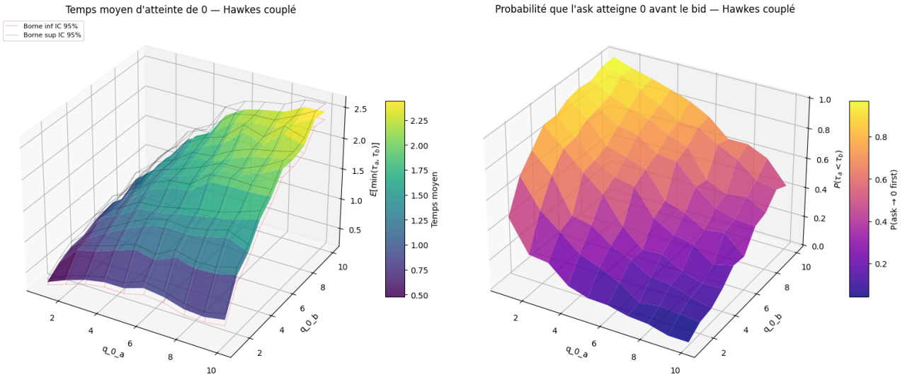
Figure 10 – Surfaces 3D pour le Hawkes couplé. Gauche : \mathbb{E}[\min(\tau_a, \tau_b)] avec IC 95%. Droite : \mathbb{P}(\tau_a < \tau_b) . Axes x, y : q_{0,a}^a, q_{0,b}^b .
