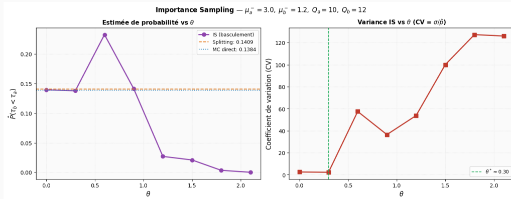
Figure 22 — Gauche : estimation de P(\tau_b < \tau_a) en fonction de \theta , comparée aux références AMS et MC direct. Droite : coefficient de variation empirique de l'IS. Horiz. : \theta ; vert. : probabilité / CV.
