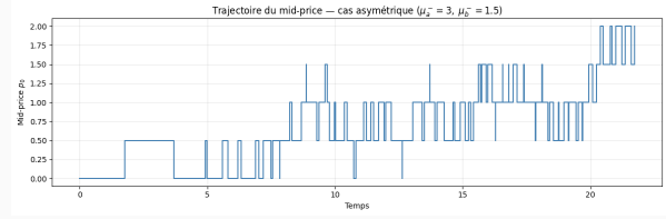
(b) Cas asymétrique. La tendance haussière est nettement visible dès les premiers cycles. Horiz. : temps ; vert. : mid-price (ticks).
