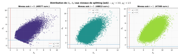
(a) États (\lambda_a^-, \lambda_b^-) aux niveaux k = 8, 5, 1 — côté ask. Les survivants ont \lambda_a^- \gg \mu_a^- = 3 . Horiz. : \lambda_a^- ; vert. : \lambda_b^- .
