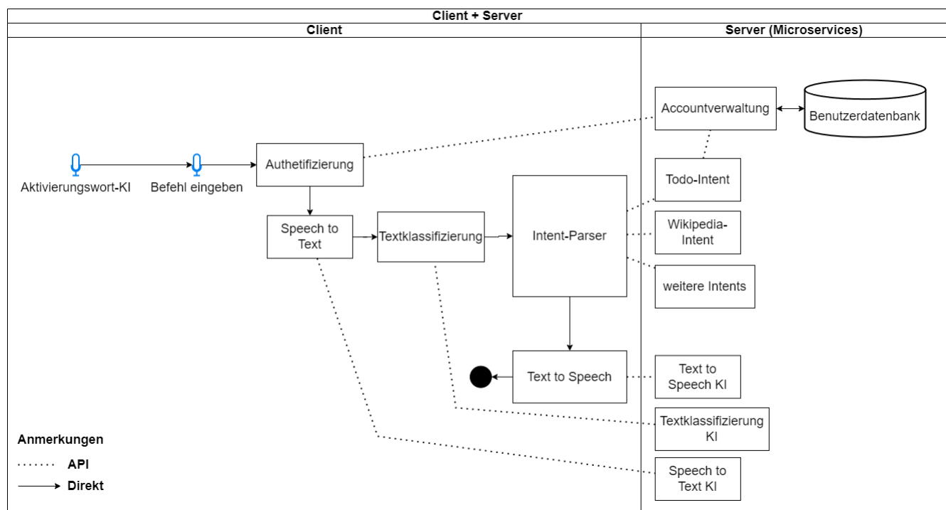
Abbildung 5. Aktivitätsdiagramm
