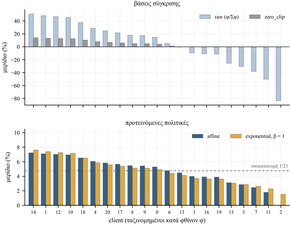
Σχήμα 5.15. Τα μερίδια κάθε client υπό τις τέσσερις πολιτικές, με τη σειρά του Σχήματος 5.3. Πάνω οι δύο βάσεις σύγκρισης και κάτω οι δύο προτεινόμενες πολιτικές, η καθεμία στη δική της κλίμακα, με τη διακεκομμένη γραμμή της ισοκατανομής. Η raw παράγει αρνητικά μερίδια, η zero_clip μηδενίζει εννέα clients, η αφινική [28] μόνο τον πιο ακραίο και η εκθετική [41] δίνει θετικό μερίδιο σε όλους.
