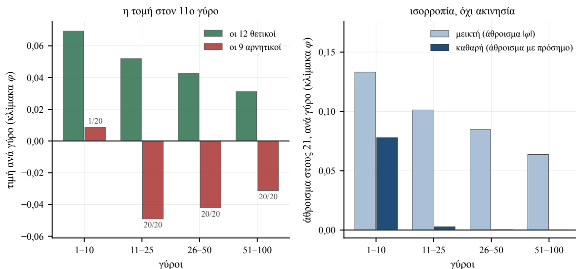
Σχήμα 5.9. Αριστερά: η τιμή ανά βαθμολογημένο γύρο, χωριστά για τις δύο ομάδες clients, μέσος όρος 20 seeds. Μέχρι τον δέκατο γύρο και οι δύο είναι θετικές. Στην άκρη κάθε στήλης των αρνητικών, το πλήθος των seeds στα οποία η ομάδα βγαίνει κάτω από το μηδέν. Δεξιά: το άθροισμα και των 21, επίσης ανά βαθμολογημένο γύρο. Το άθροισμα με πρόσημο σβήνει μετά τον δέκατο γύρο, ενώ το άθροισμα των απόλυτων τιμών όχι. Και τα δύο πάνελ δείχνουν ρυθμό ανά γύρο, ώστε οι ομάδες γύρων άνισου πλάτους να συγκρίνονται μεταξύ τους.
