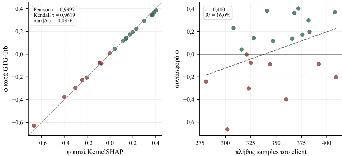
Σχήμα 5.4. Αριστερά: οι δύο εκτιμητές δίνουν ουσιαστικά την ίδια τιμή σε κάθε client. Δεξιά: ο όγκος δεδομένων εξηγεί μόνο το 16% της διακύμανσης της συνεισφοράς. Κόκκινα τα σημεία με αρνητικό \varphi .
