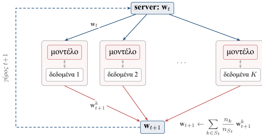
Σχήμα 2.1. Ένας γύρος. Ο server εκπέμπει το global model, κάθε client το εκπαιδεύει E εποχές πάνω στα δικά του δεδομένα και επιστρέφει μόνο τις παραμέτρους. Τα δεδομένα δε βγαίνουν ποτέ από το πλαίσιο του client. Ο σταθμισμένος μέσος δίνει το μοντέλο του επόμενου γύρου.
