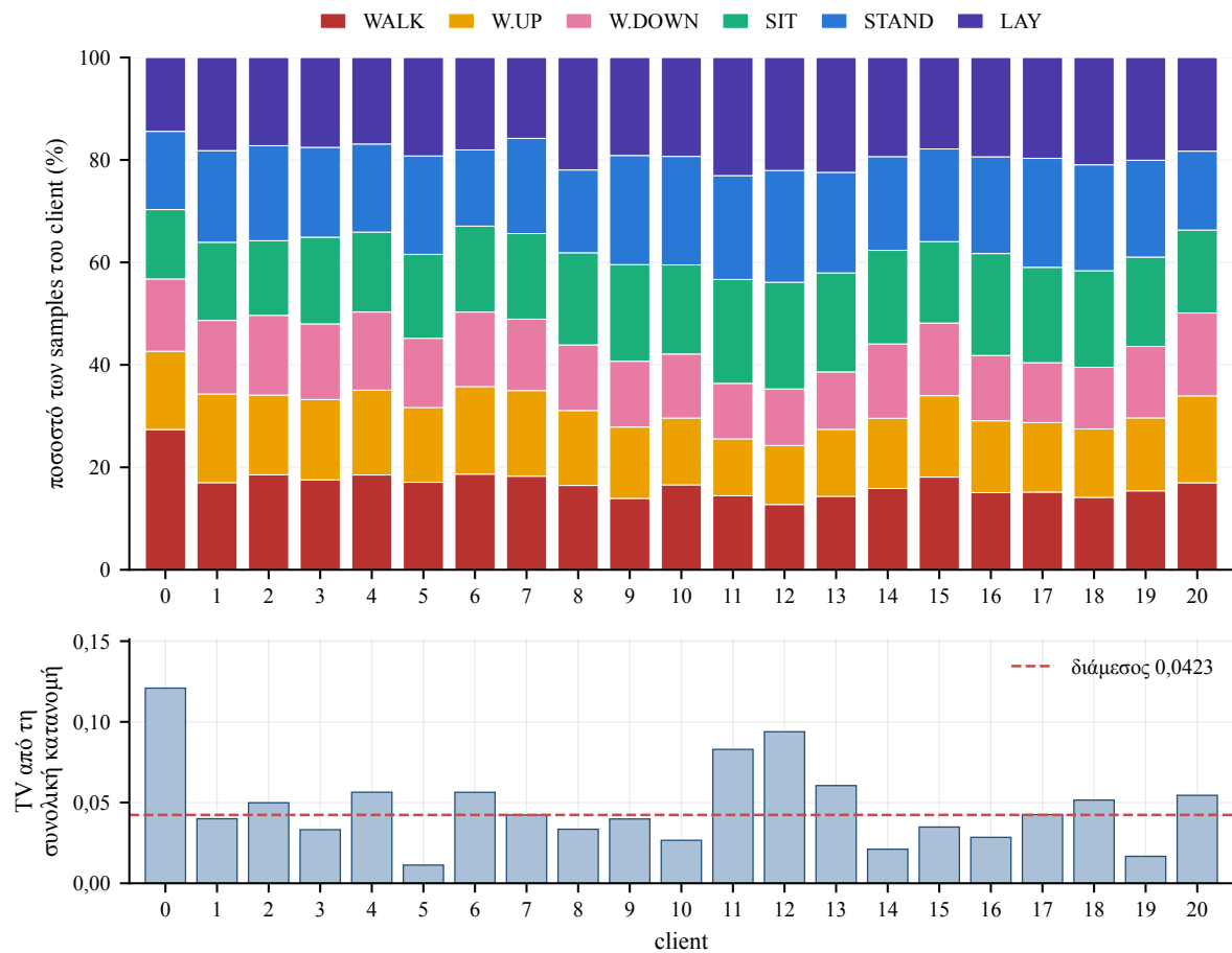
Σχήμα 3.2. Πάνω: η σύνθεση των δεδομένων κάθε client ανά δραστηριότητα. Κάτω: η απόσταση ολικής μεταβολής της κατανομής του καθενός από τη συνολική. Καμία κλάση δε λείπει από κανέναν. Η διάμεση απόσταση είναι 0,0423.
