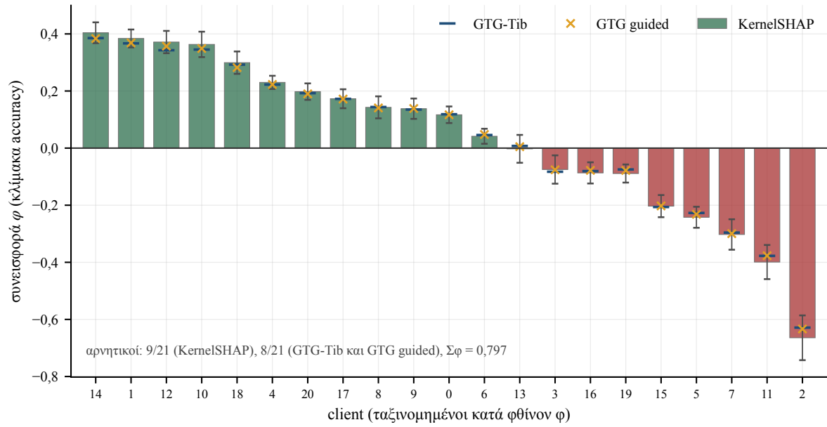
Σχήμα 5.3. Η συνεισφορά \varphi κάθε client, σε μονάδες ορθότητας, μέσος όρος 20 seeds. Οι μπάρες είναι ο εκτιμητής KernelSHAP με \pm μία τυπική απόκλιση μεταξύ seeds, ενώ οι οριζόντιες παύλες είναι το GTG-Tib και τα σταυρουδάκια η πλήρης εκδοχή με καθοδηγούμενη δειγματοληψία (GTG guided). Οι δύο εκτιμητές μεταθέσεων δίνουν 8 αρνητικούς αντί για 9, γιατί διαφωνούν μόνο στον client 13, που είναι ο μόνος με τιμή μέσα στον θόρυβο.
