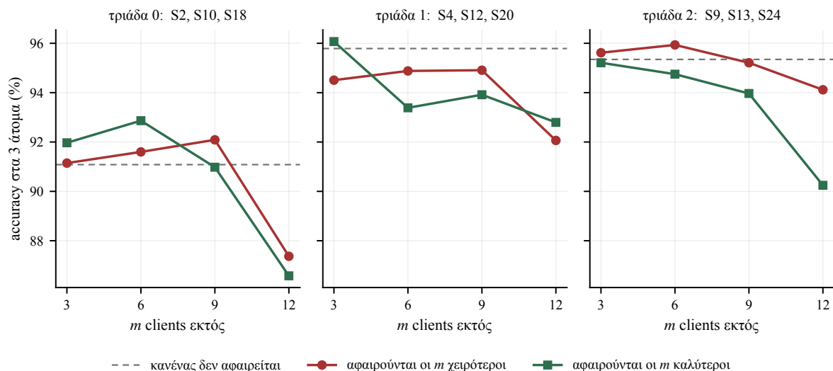
Σχήμα 5.14. Ορθότητα στα τρία άτομα που κρατήθηκαν έξω από την απόφαση, όταν αφαιρούνται οι m χειρότεροι ή οι m καλύτεροι clients. Η διακεκομμένη γραμμή είναι η ορθότητα χωρίς καμία αφαίρεση. Όπου η πράσινη καμπύλη βρίσκεται πάνω από την κόκκινη, η αφαίρεση των καλύτερων ωφέλησε περισσότερο από την αφαίρεση των χειρότερων.
