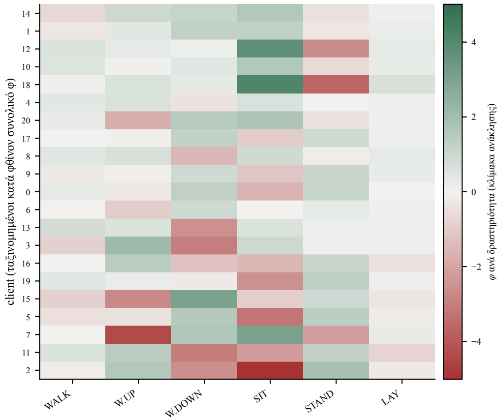
Σχήμα 5.10. Η συνεισφορά κάθε client σε κάθε δραστηριότητα, σε μονάδες ανάκλισης. Οι γραμμές είναι ταξινομημένες κατά φθίνον συνολικό \varphi . Πράσινο σημαίνει θετική και κόκκινο αρνητική συνεισφορά, όπως στο Σχήμα 5.3.
