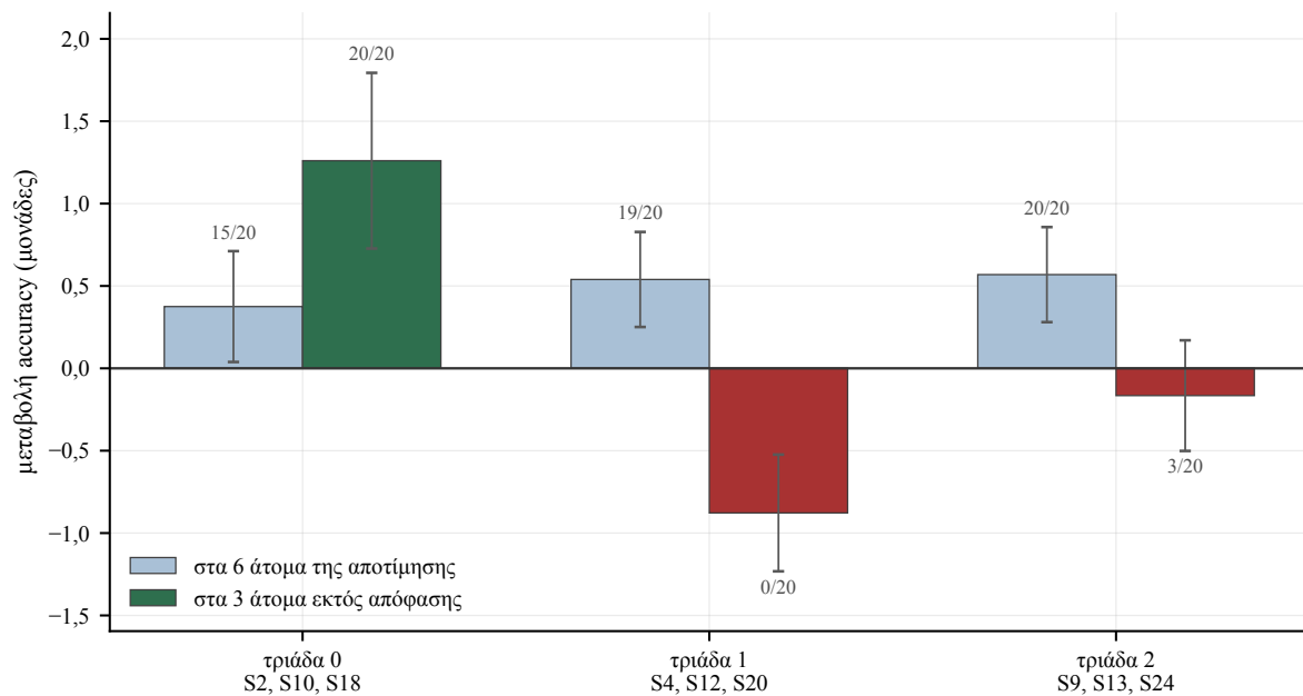
Σχήμα 5.13. Η επίδραση της αφαίρεσης, μέσος όρος 20 seeds, με τυπική απόκλιση μεταξύ seeds. Οι ανοιχτές γαλάζιες στήλες μετρούν στα έξι άτομα με τα οποία έγινε η αποτίμηση και είναι θετικές και στις τρεις τριάδες. Οι έγχρωμες μετρούν στα τρία άτομα που κρατήθηκαν έξω από κάθε απόφαση και αλλάζουν πρόσημο, πράσινες όπου η αφαίρεση βοηθά και κόκκινες όπου βλάπτει. Στην άκρη κάθε στήλης, το πλήθος των seeds με θετικό πρόσημο.
