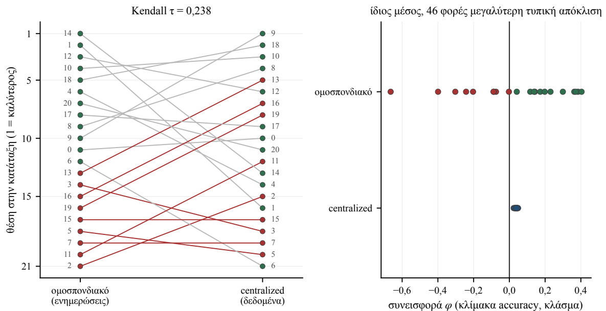
Σχήμα 5.8. Αριστερά: η θέση κάθε client στο ομοσπονδιακό παίγνιο και στο παίγνιο επανεκπαίδευσης του κεντρικού μοντέλου (centralized στο σχήμα). Με κόκκινο όσοι λαμβάνουν αρνητική τιμή στο ομοσπονδιακό. Δεξιά: οι δύο κατανομές των \varphi στον ίδιο άξονα. Το άθροισμα και ο μέσος είναι ουσιαστικά ταυτόσημα, η διασπορά όχι.
