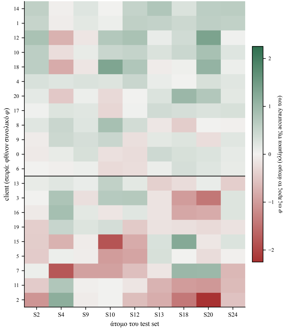
Σχήμα 5.11. Η μήτρα 21 \times 9 με τη συνεισφορά κάθε client προς κάθε άτομο του συνόλου ελέγχου, εκτιμητής KernelSHAP, μέσοι όροι 20 seeds. Οι clients είναι ταξινομημένοι κατά φθίνον συνολικό \varphi , όπως στο Σχήμα 5.3. Η οριζόντια γραμμή χωρίζει τους 12 θετικούς από τους 9 αρνητικούς. Πράσινο σημαίνει θετική και κόκκινο αρνητική συνεισφορά, όπως στα Σχήματα 5.3 και 5.10. Καμία γραμμή κάτω από τη γραμμή διαχωρισμού δεν είναι ολόκληρη κόκκινη.
