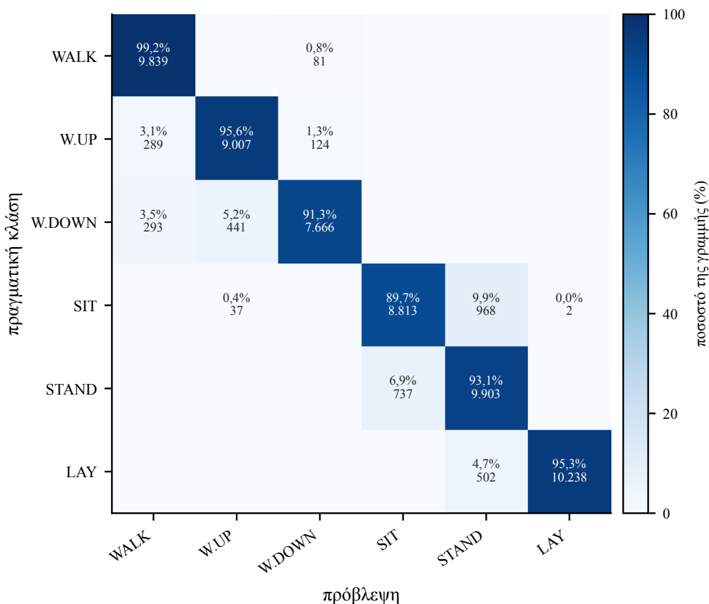
Σχήμα 4.6. Άθροισμα 20 seeds, 58.940 προβλέψεις. Κάθε κελί δείχνει το ποσοστό της γραμμής και το απόλυτο πλήθος. Το ζεύγος SITTING και STANDING συγκεντρώνει σχεδόν τα μισά σφάλματα του μοντέλου.
