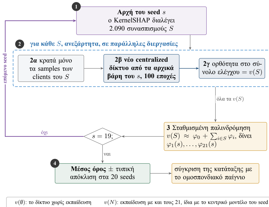
Σχήμα 5.7. Η αποτίμηση στο παίγνιο επανεκπαίδευσης. Το βήμα 2 γίνεται μία φορά για κάθε συνασπισμό και είναι το μόνο που εκπαιδεύει, πάντα ένα centralized μοντέλο με τα δεδομένα των clients του συνασπισμού. Κάθε seed έχει ένα μόνο παίγνιο, οπότε η τιμή του seed βγαίνει κατευθείαν από την παλινδρόμηση.
