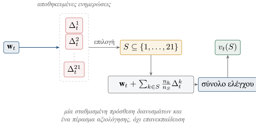
Σχήμα 5.1. Η αποτίμηση της v_t(S) . Οι ενημερώσεις όλων των clients αποθηκεύονται μία φορά ανά γύρο. Κάθε συνασπισμός ανασυντίθεται από αυτές με σταθμισμένη πρόσθεση και αποτιμάται με ένα πέρασμα αξιολόγησης. Η πλήρης επανεκπαίδευση, που θα απαιτούσε 2^{21} ομοσπονδιακές εκπαιδεύσεις ανά seed, αποφεύγεται.
