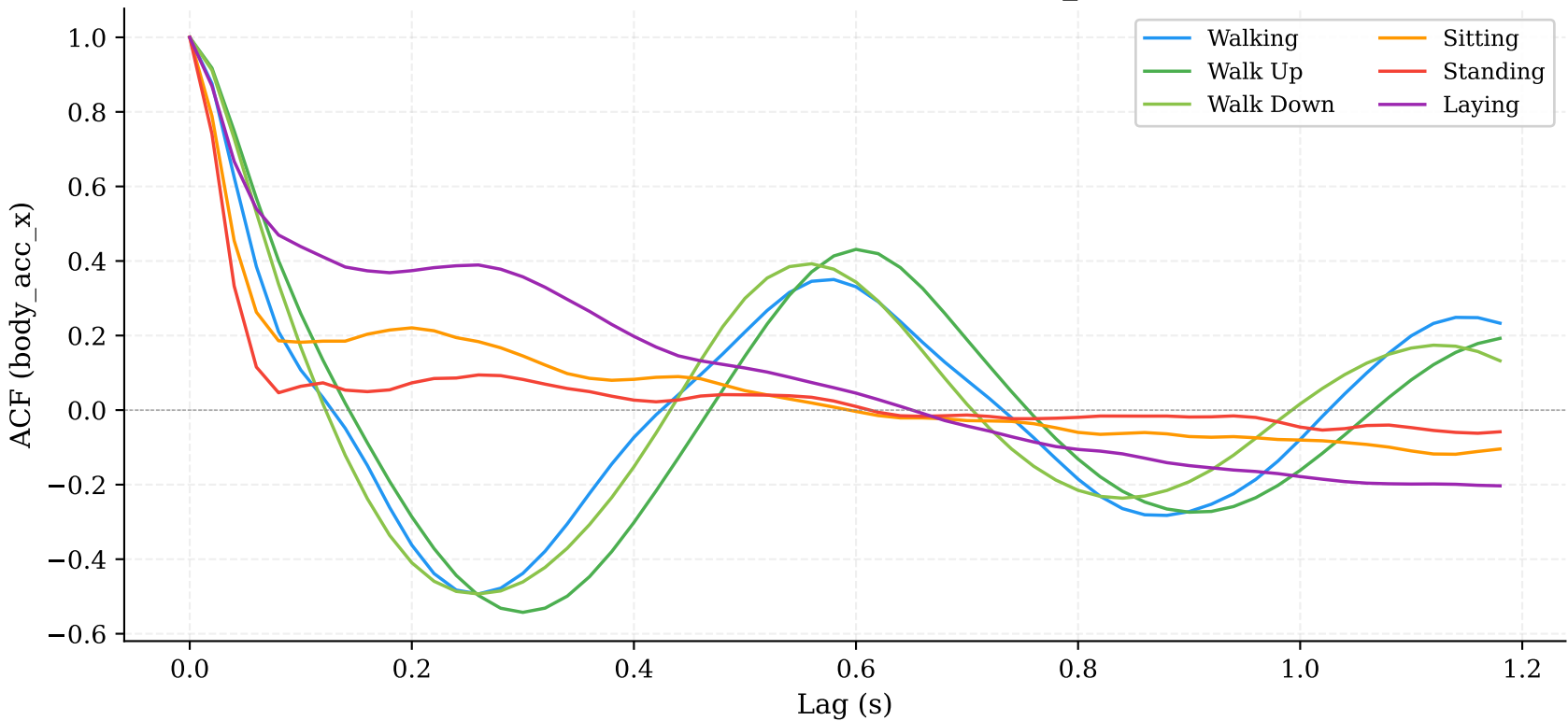
Autocorrelation ανά κλάση — UCI_HAR
