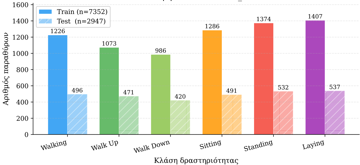
Κατανομή κλάσεων — UCI_HAR
