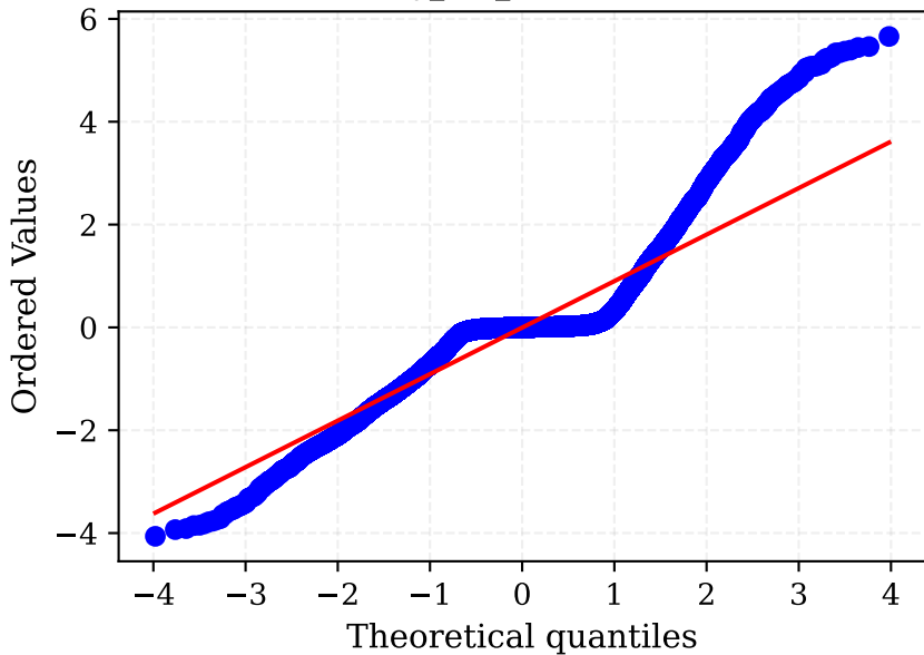
body_acc_x (Q-Q plot)
