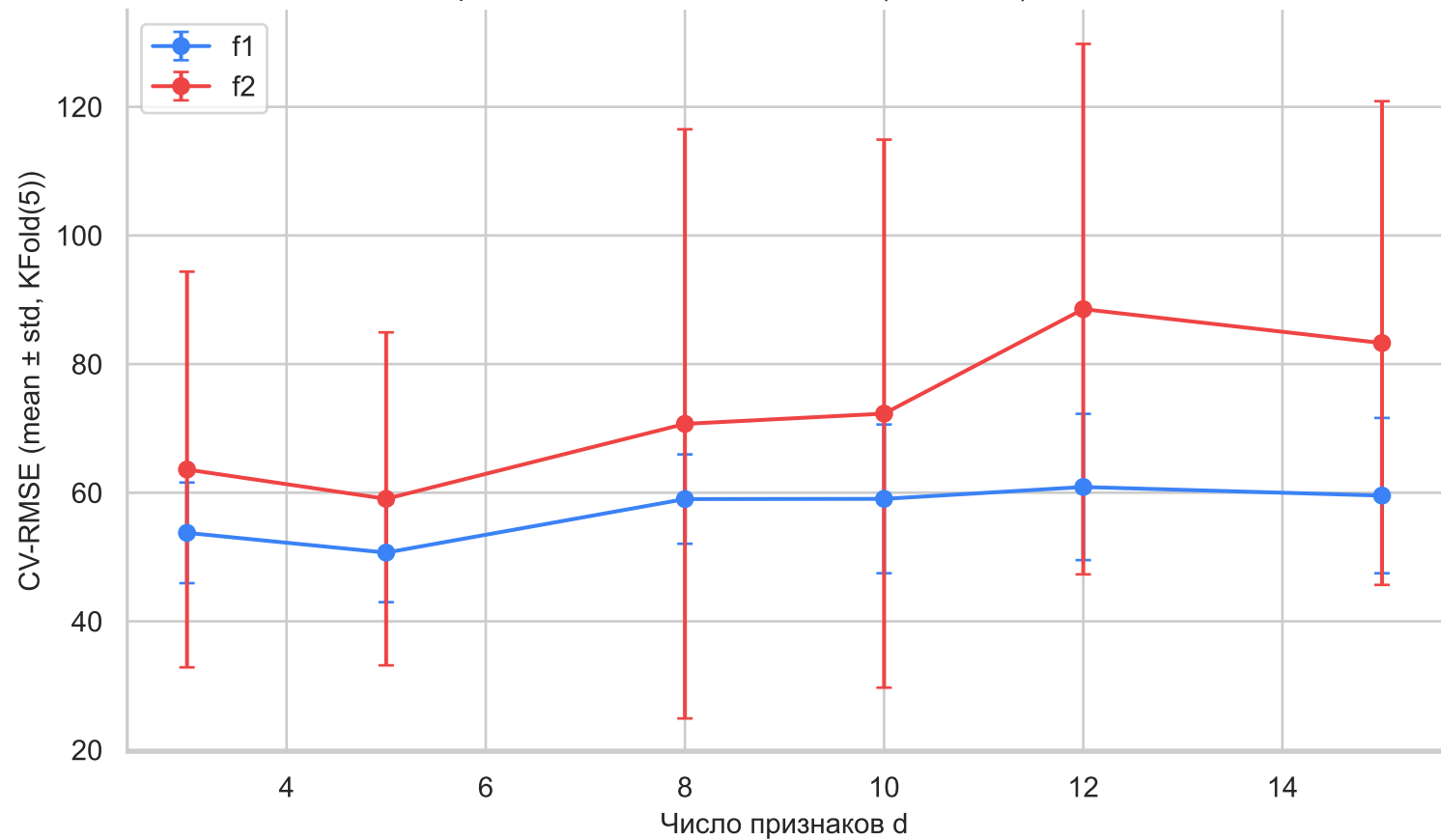
Кривая d \rightarrow \text{CV-RMSE} для NW(Gaussian) — dau
