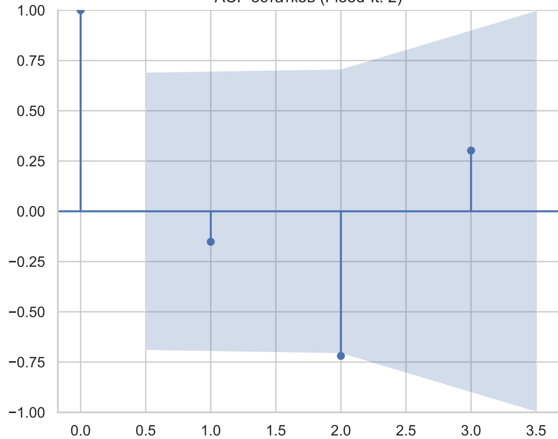
ACF остатков (Flood-It! 2)
