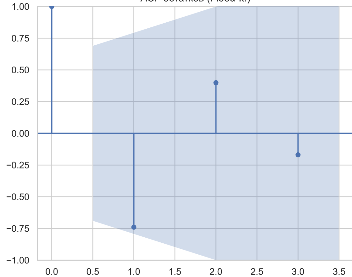
ACF остатков (Flood-It!)
