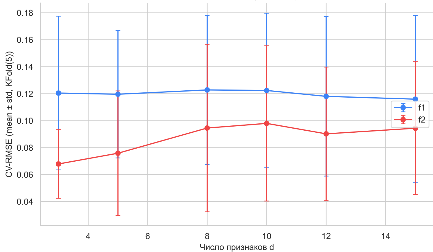
Кривая d \rightarrow \text{CV-RMSE} для NW(Gaussian) — stickiness
