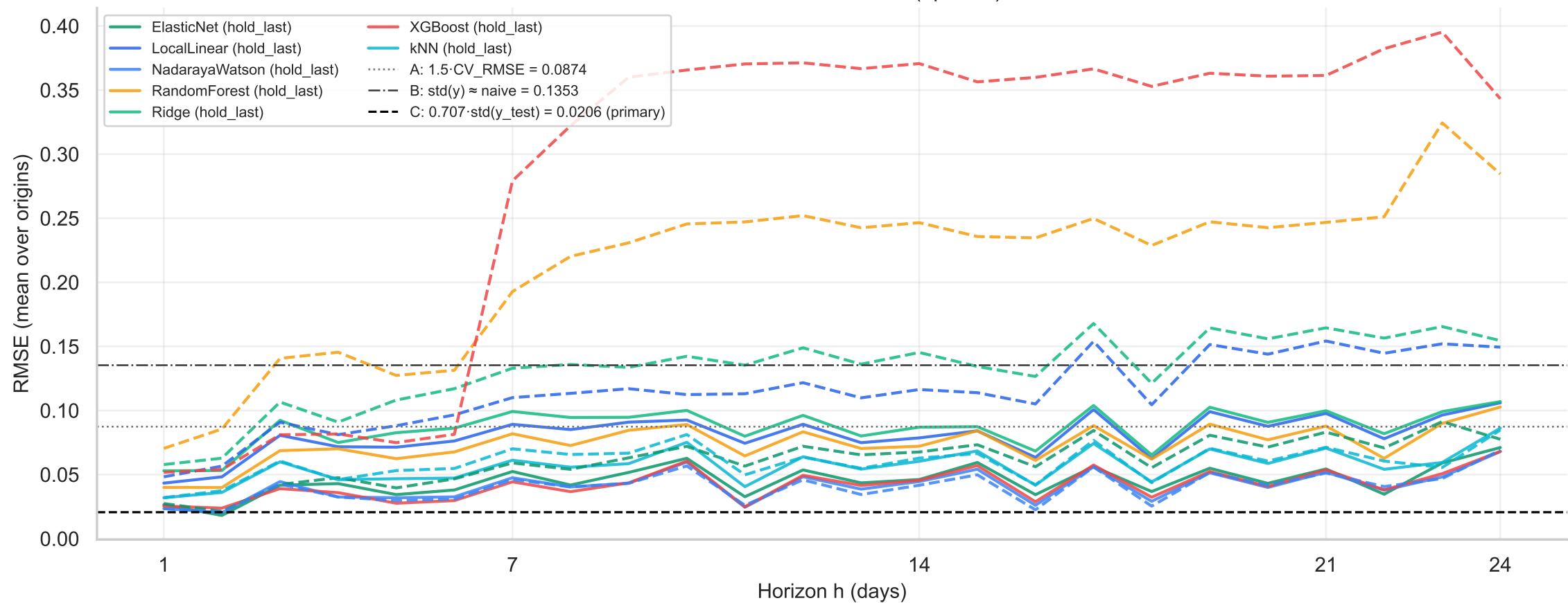
Forecast horizon curve — Flood-It! 2 (провал) / stickiness
