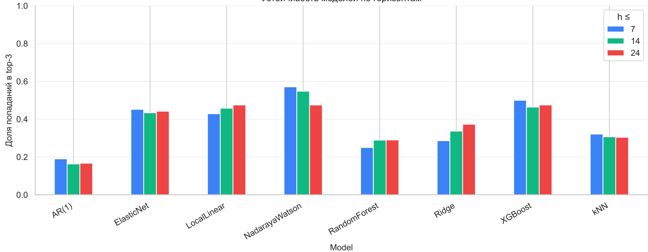
Устойчивость моделей по горизонтам
