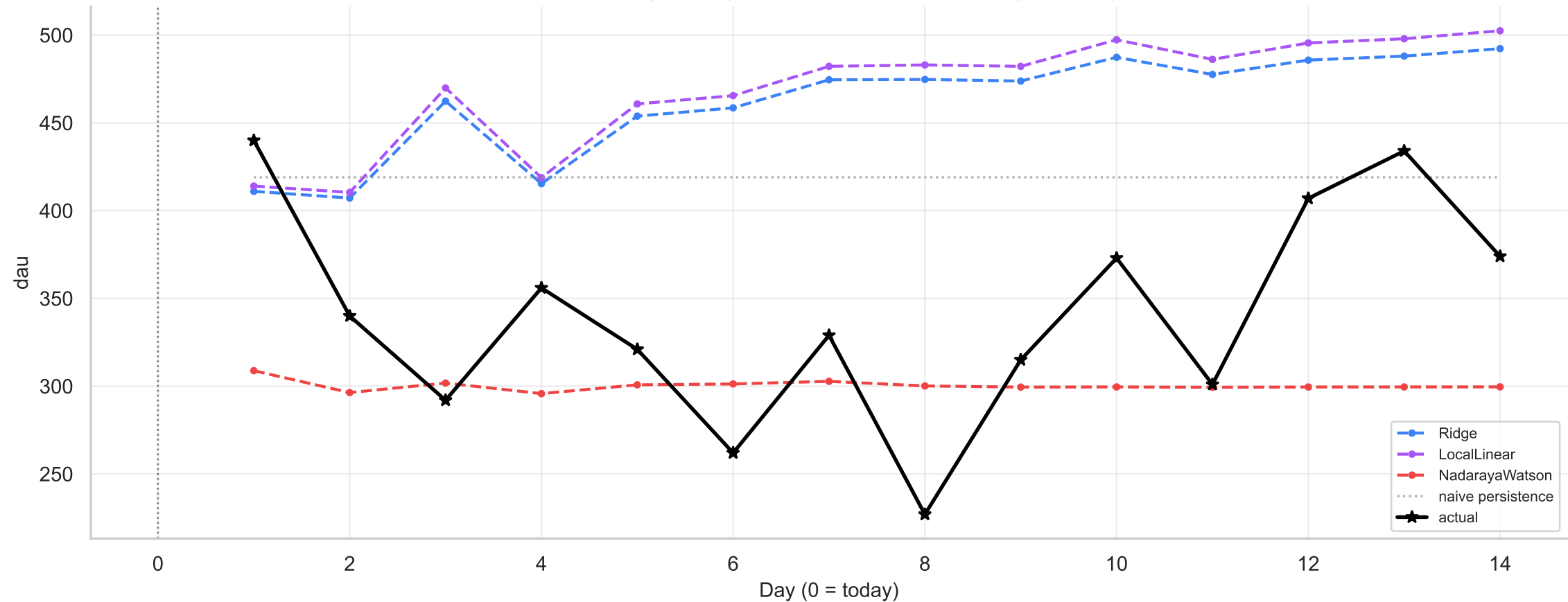
Flood-It! 2 (провал) / dau — model comparison (recursive)
