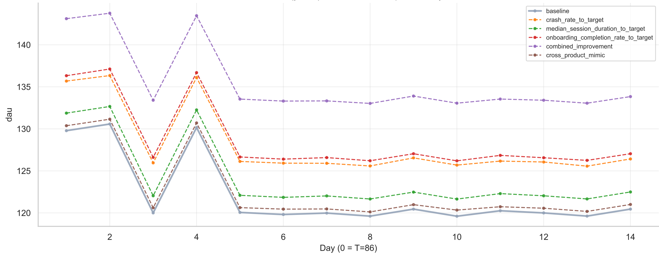
Flood-It! (успех) / dau - все сценарии overlay
