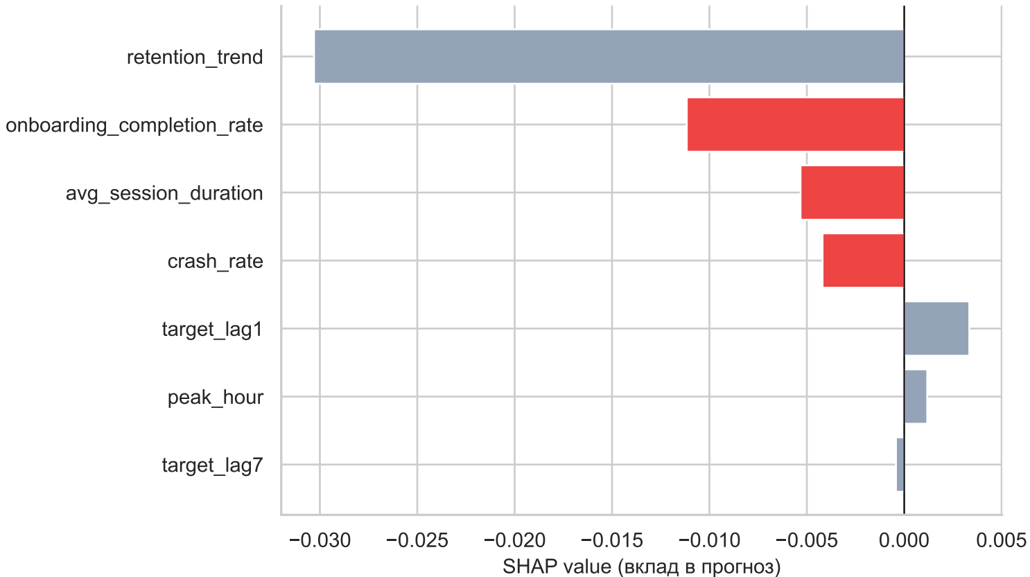
Flood-It! 2 (провал) / retention_d7 - SHAP вклады при baseline (T=86) baseline prediction = 0.0803
