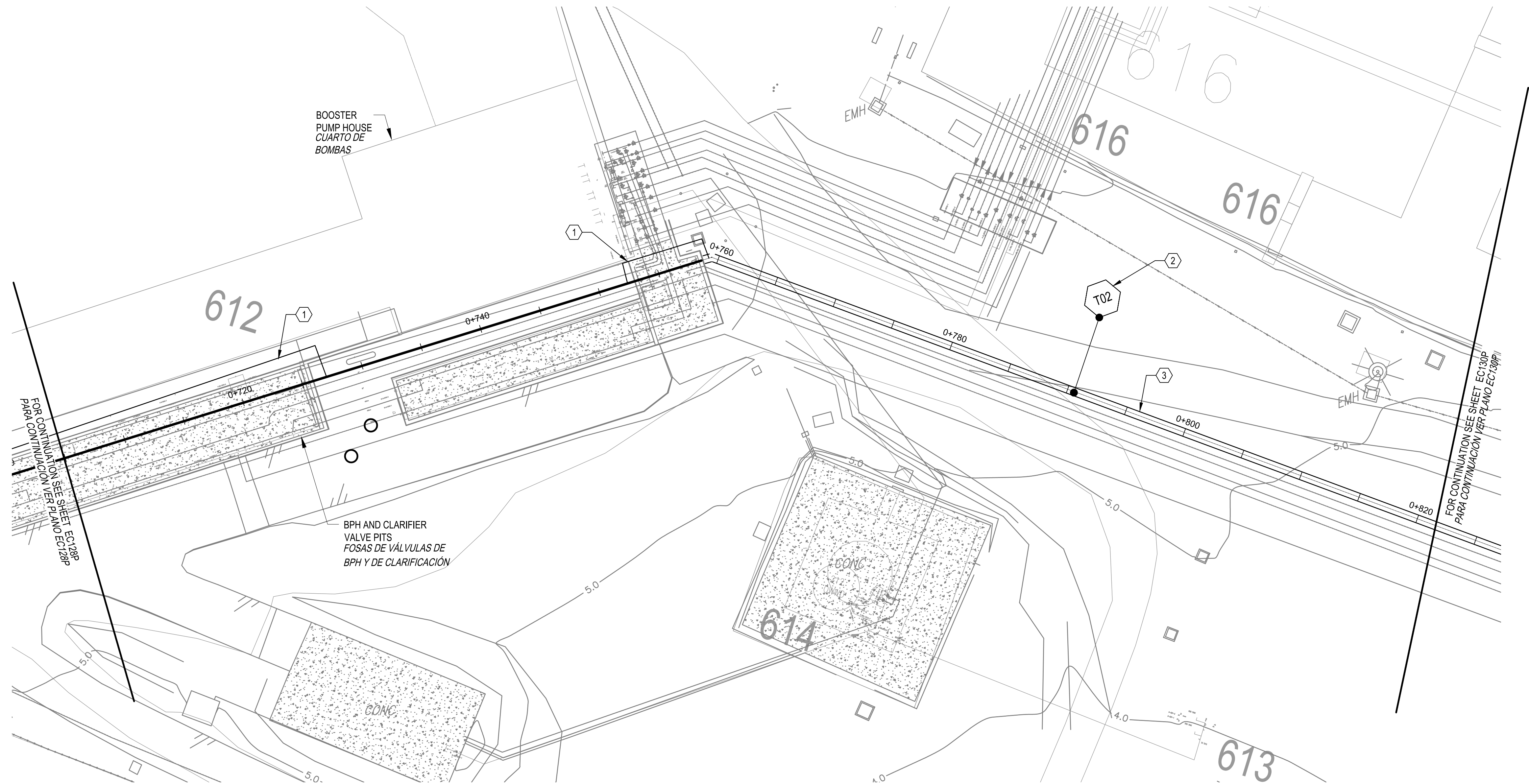
B1 CATHODIC PROTECTION PLAN PLANTA DE PROTECCIÓN CATÓDICA 1:200
