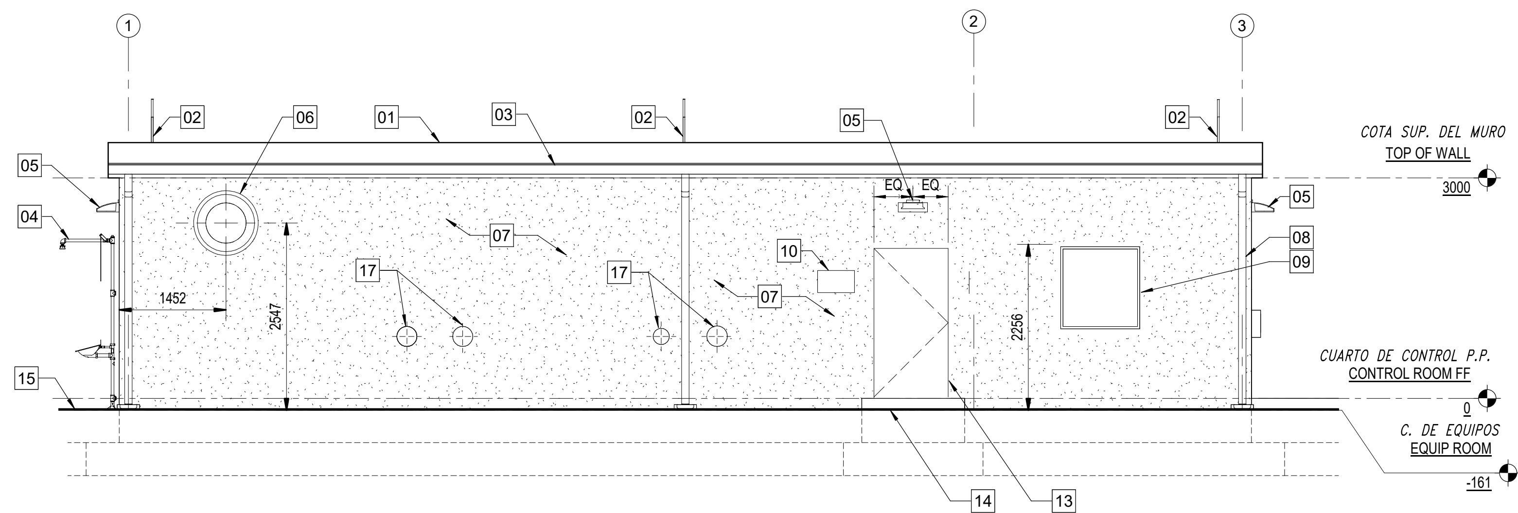
SOUTH ELEVATION ALZADO SUR SCALE: 1 : 50 ESCALA: 1 : 50
