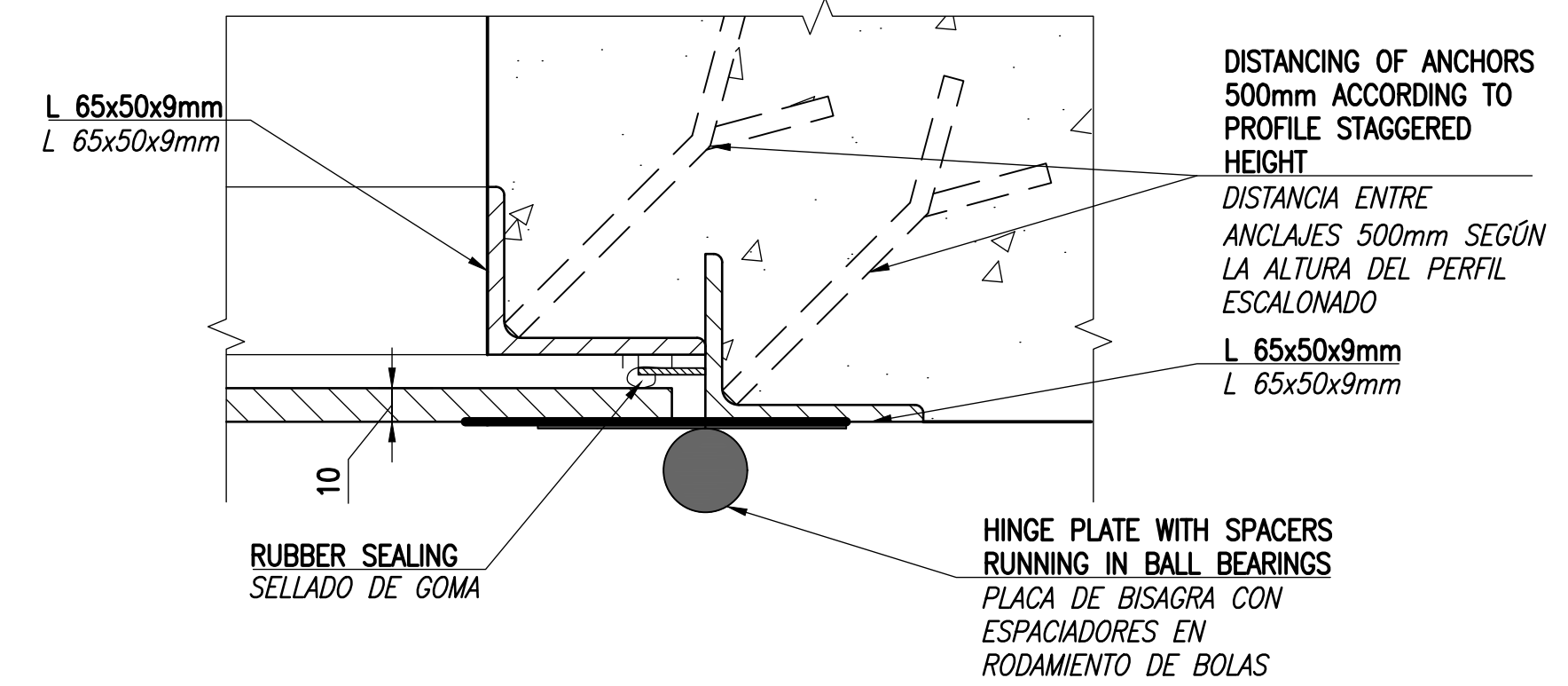
C4 HINGE DETAIL DETALLE DE BISAGRA SCALE: 1:2 ESCALA: 1:2
