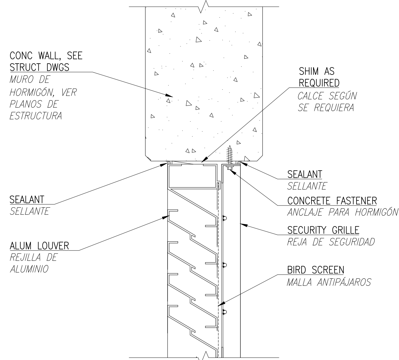
LOUVER DETAIL DETALLE DE REJILLA
