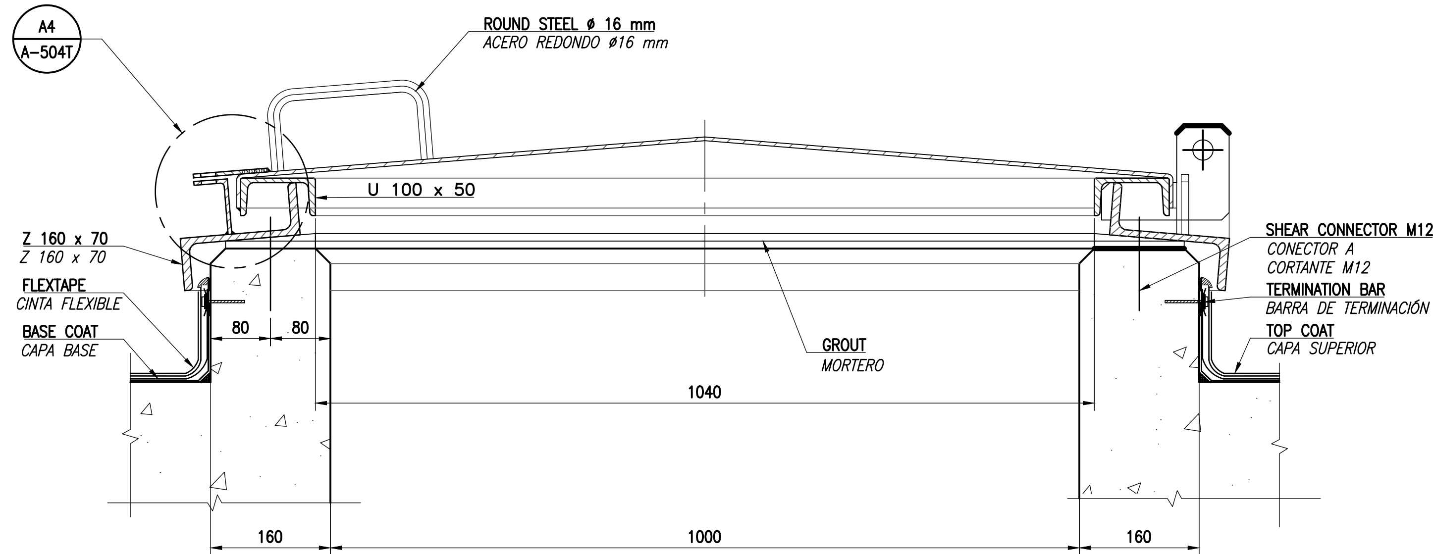
C1 SECTION SECCIÓN SCALE: 1:5 ESCALA: 1:5
