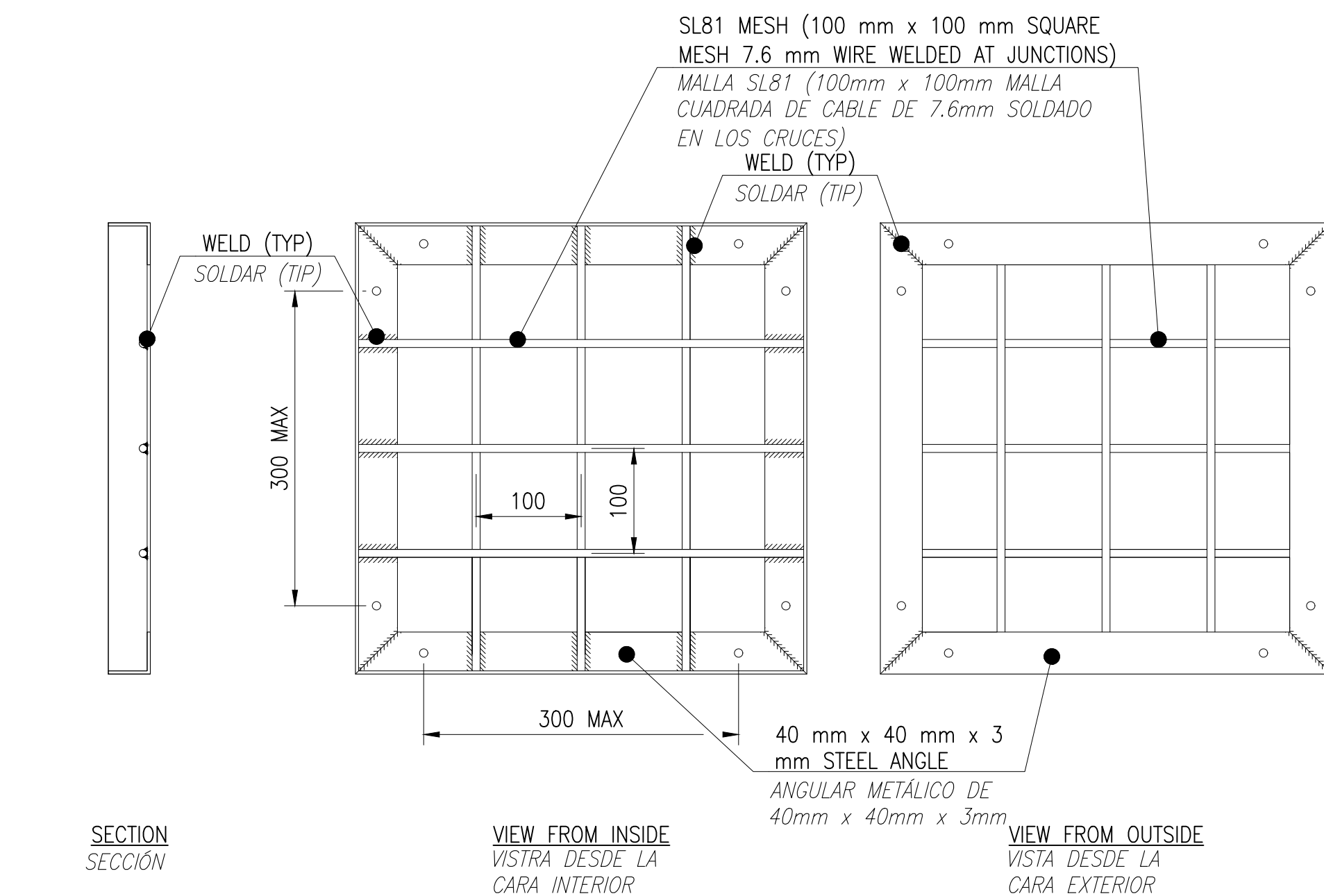
SECURITY GRILLE DETAIL DETALLE DE REJA DE SEGURIDAD
