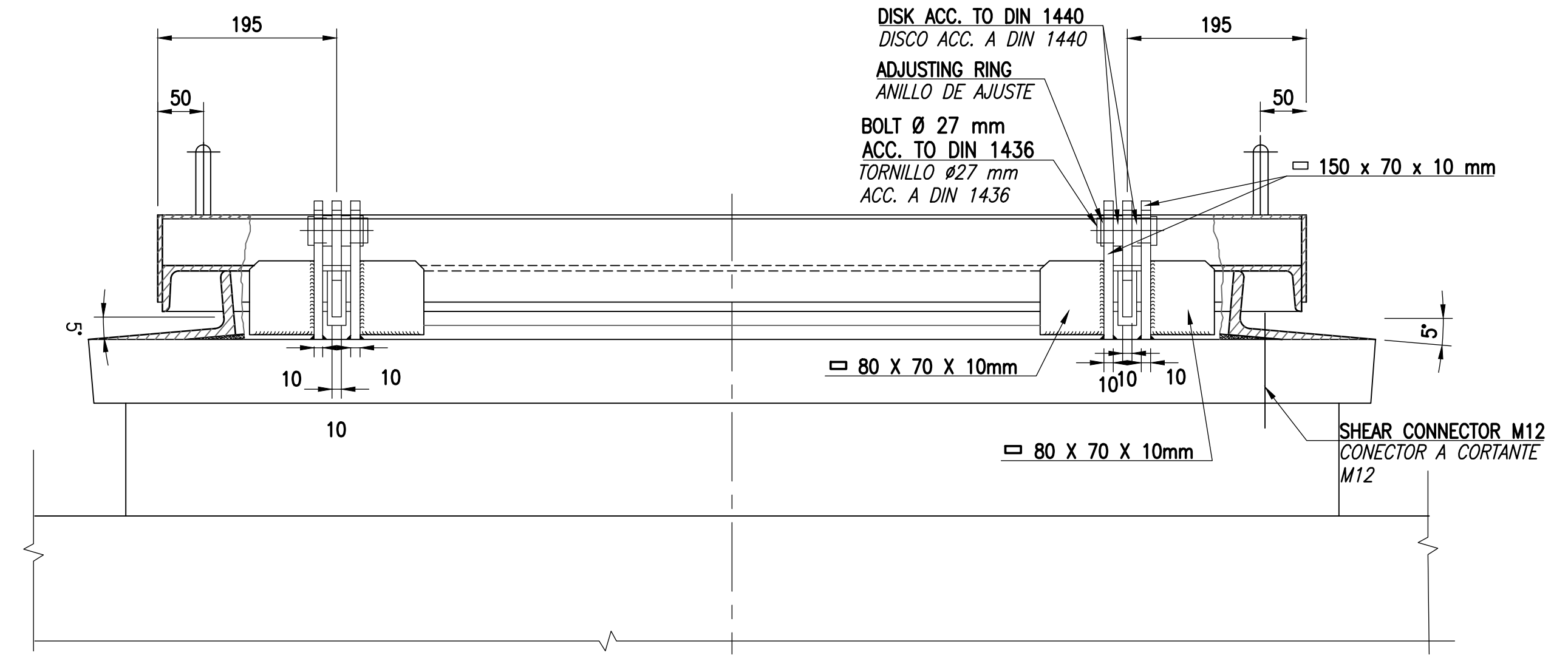
C4 SECTION SECCIÓN SCALE: 1:5 ESCALA: 1:5
