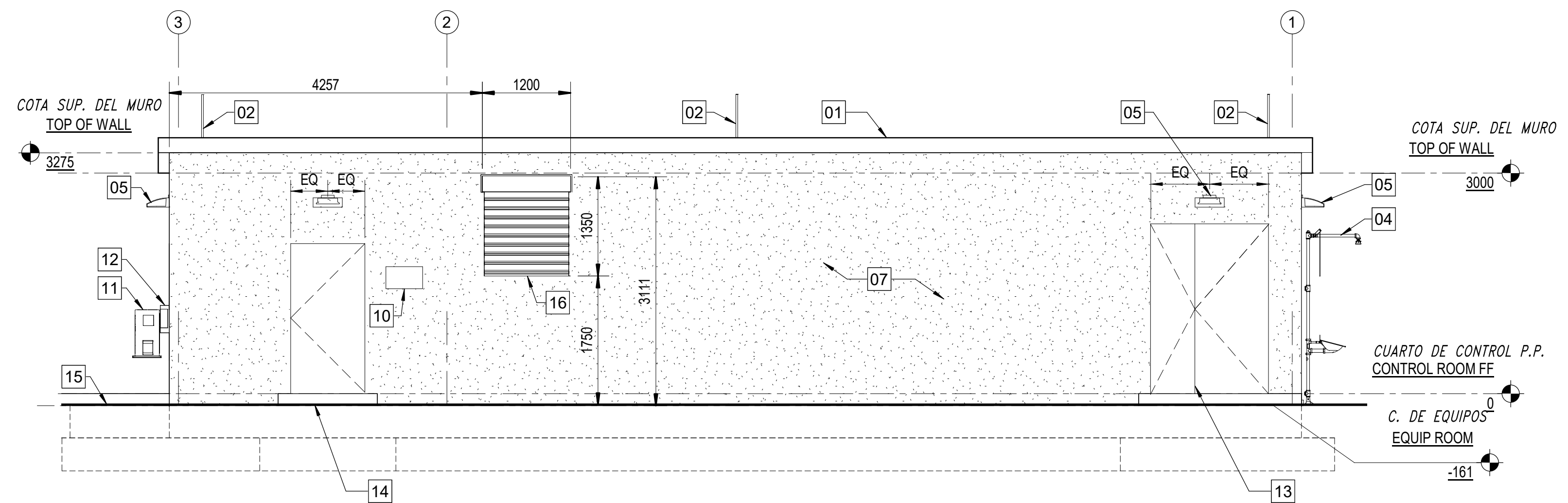
NORTH ELEVATION ALZADO NORTE SCALE: 1:50 ESCALA: 1:50
