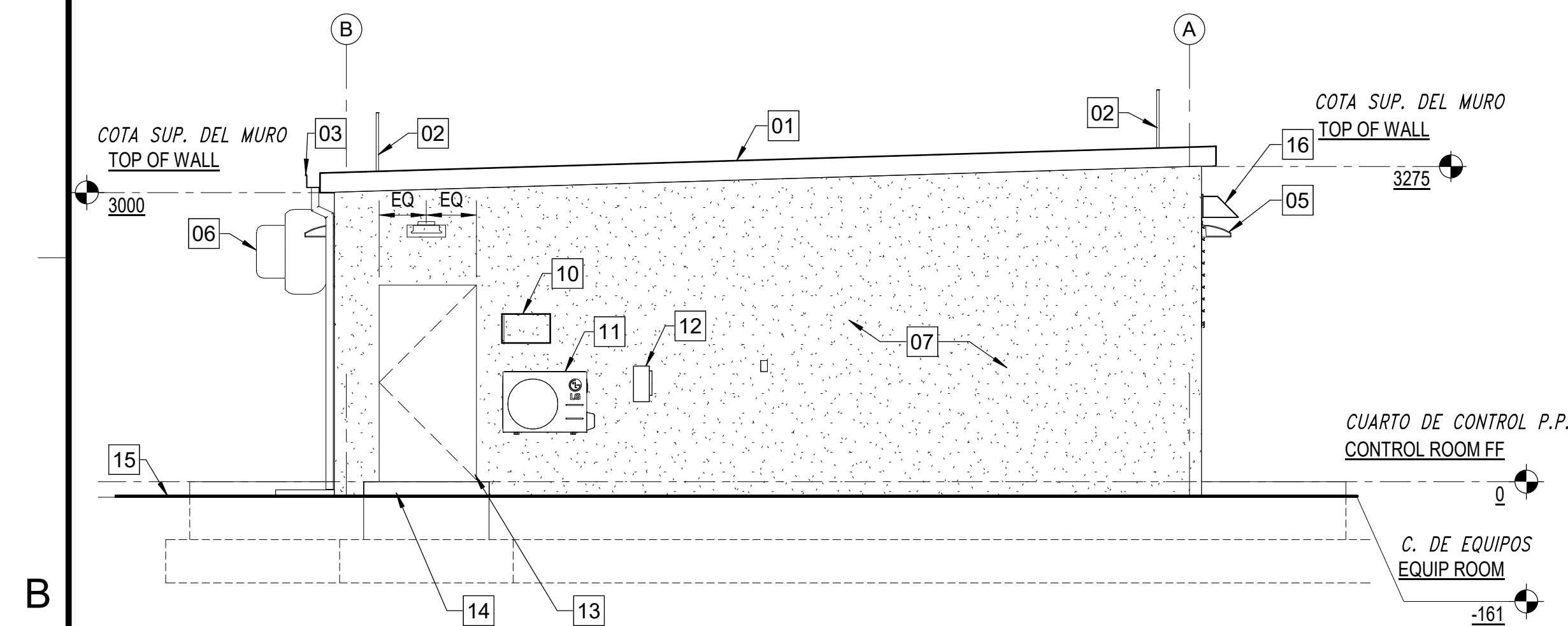
B1 EAST ELEVATION ALZADO ESTE SCALE: 1:50 ESCALA: 1:50
