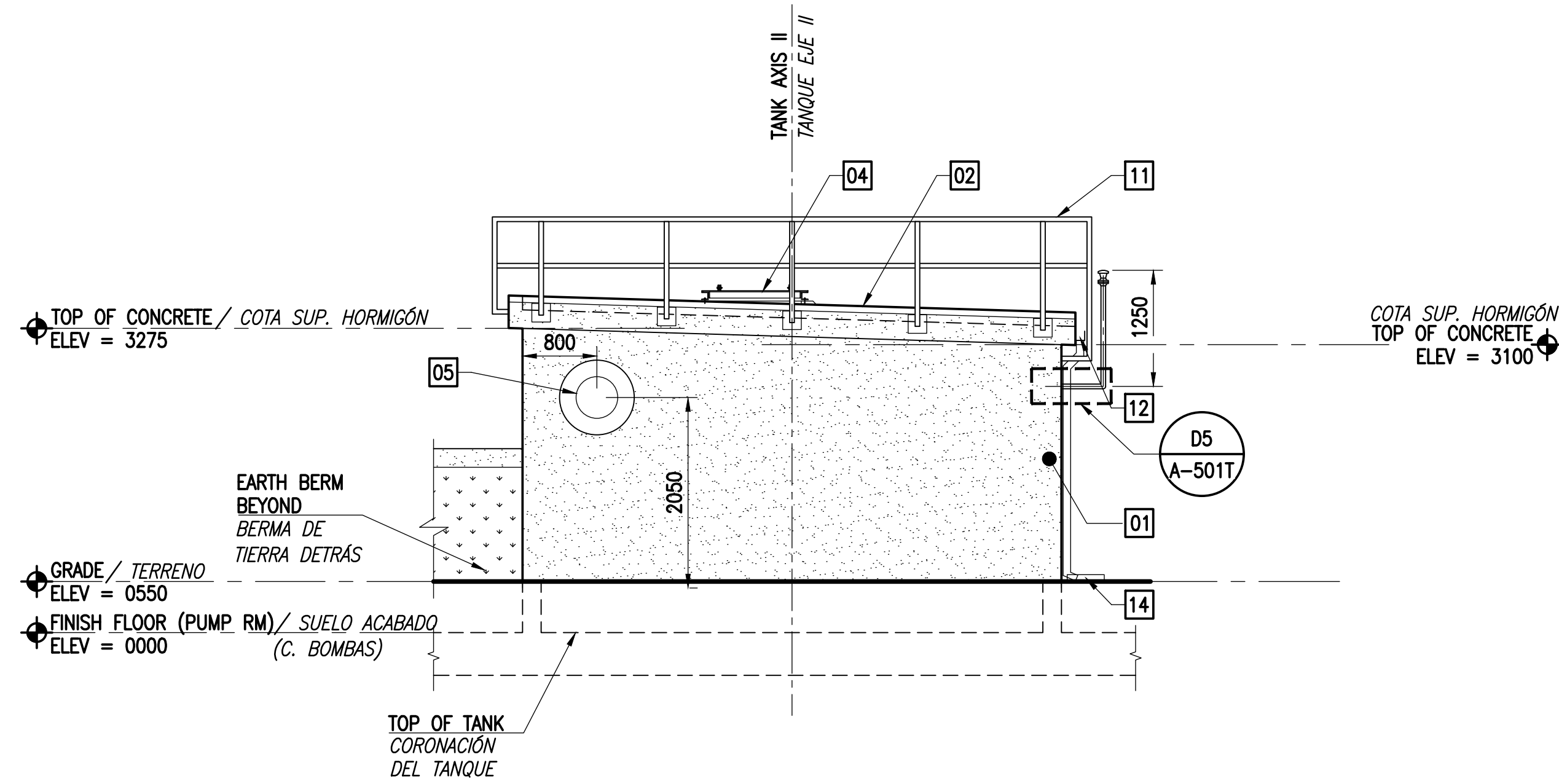
C4 ELEVATION PUMP VAULT / ALZADO CÁMARA DE BOMBAS SCALE: 1:50
