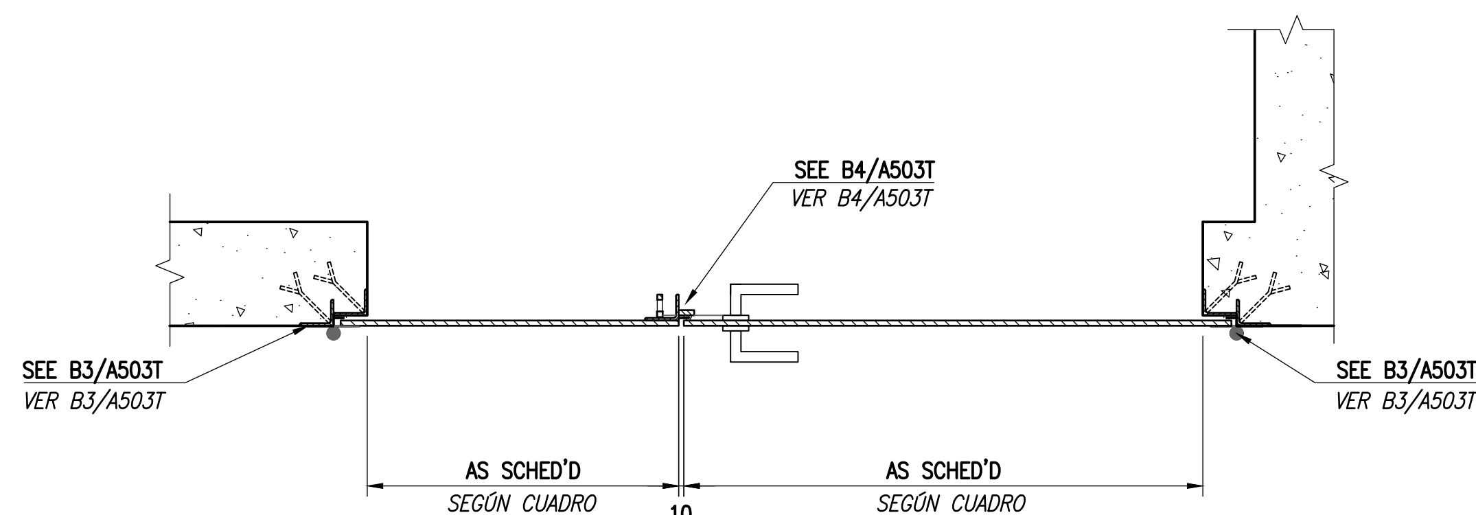
DETAIL DETALLE A3 SCALE: 1:10 ESCALA: 1:10
