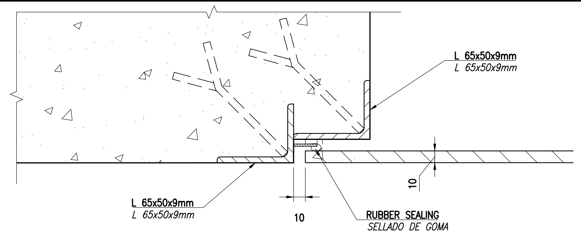
D4 LATCH DETAIL DETALLE DEL CIERRE SCALE: 1:2 ESCALA: 1:2
