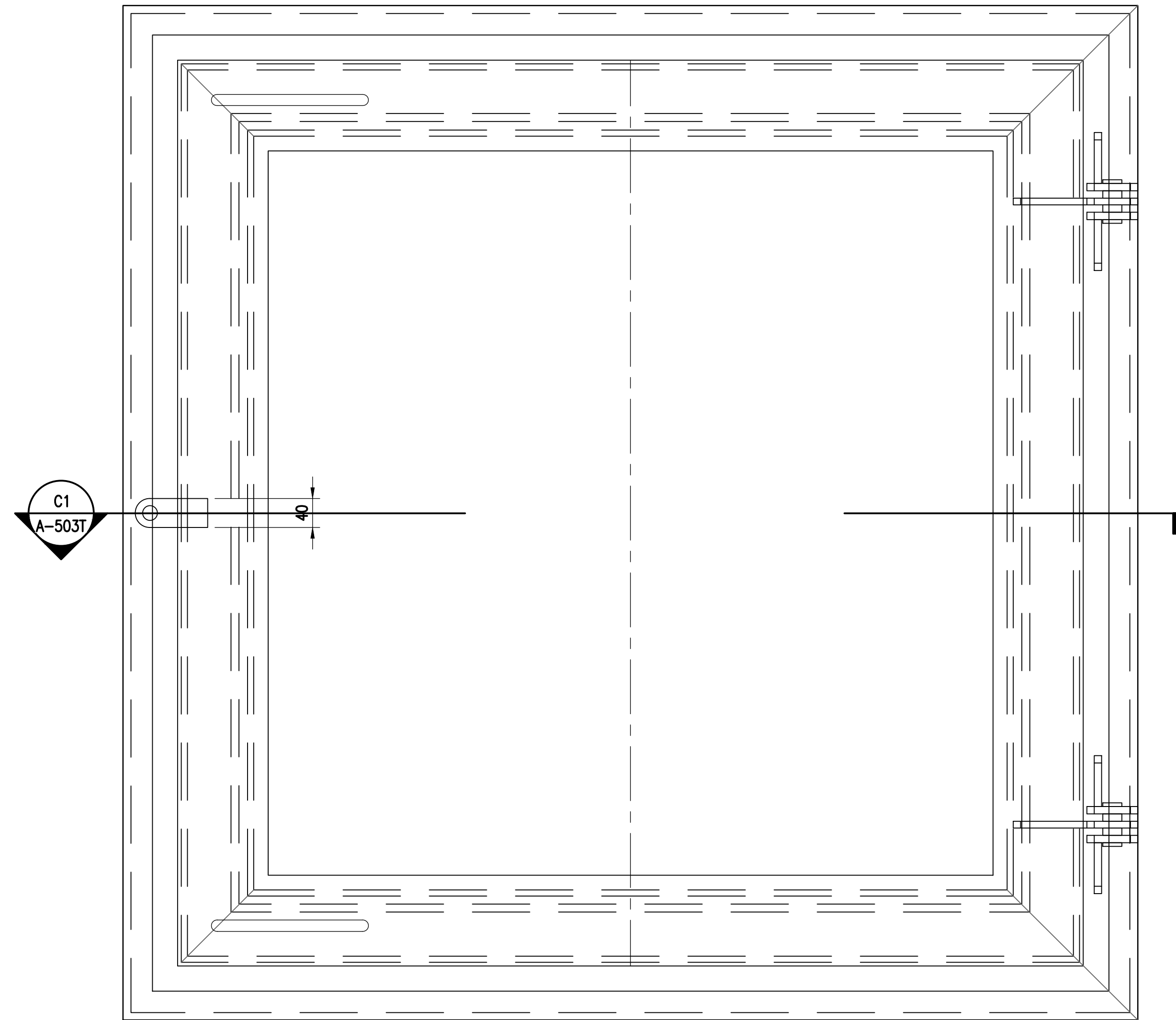
A1 PLAN VIEW VISTA EN PLANTA SCALE: 1:5 ESCALA: 1:5
