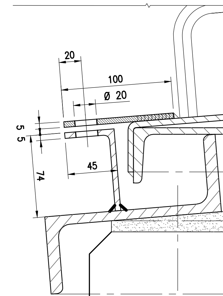
A4 DETAIL DETALLE SCALE: 1:2 ESCALA: 1:2
