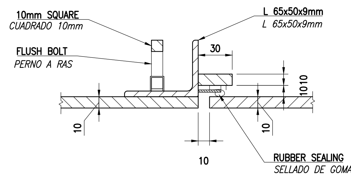
B4 ASTRAGAL DETAIL DETALLE DE ASTRÁGALO SCALE: NONE ESCALA: NINGUNA
