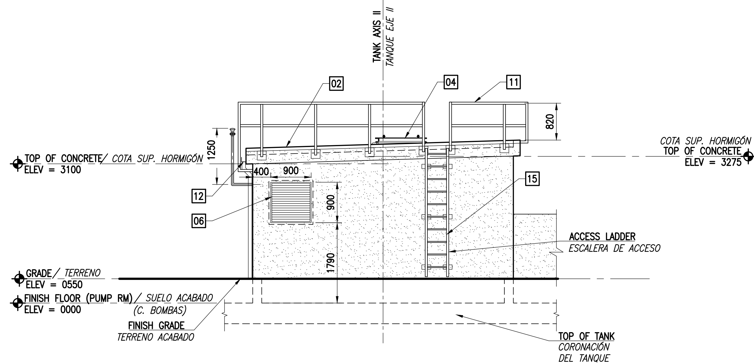
B4 ELEVATION PUMP VAULT / ALZADO CÁMARA DE BOMBAS SCALE: 1:50
