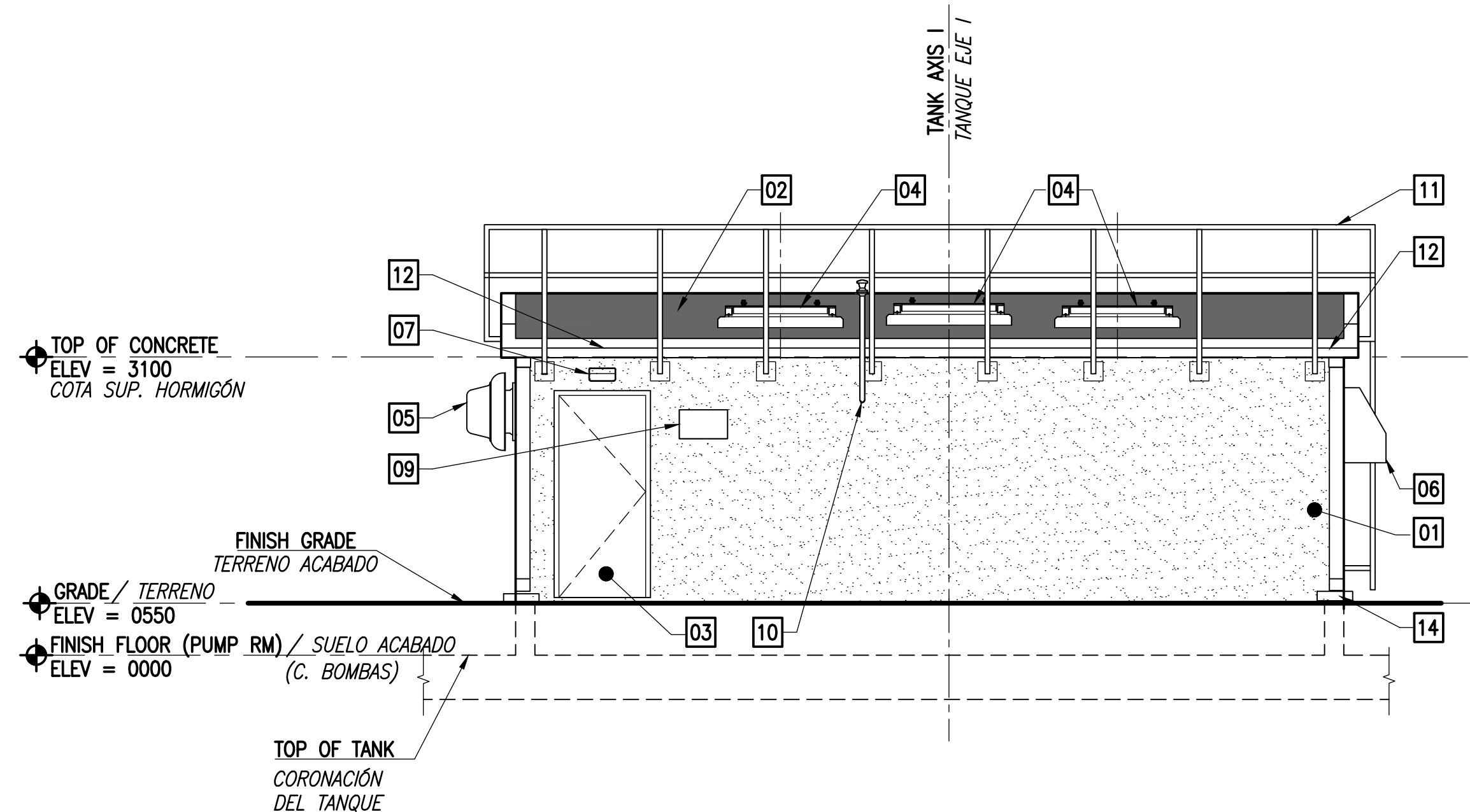
C1 ELEVATION PUMP VAULT / ALZADO CÁMARA DE BOMBAS SCALE: 1:50
