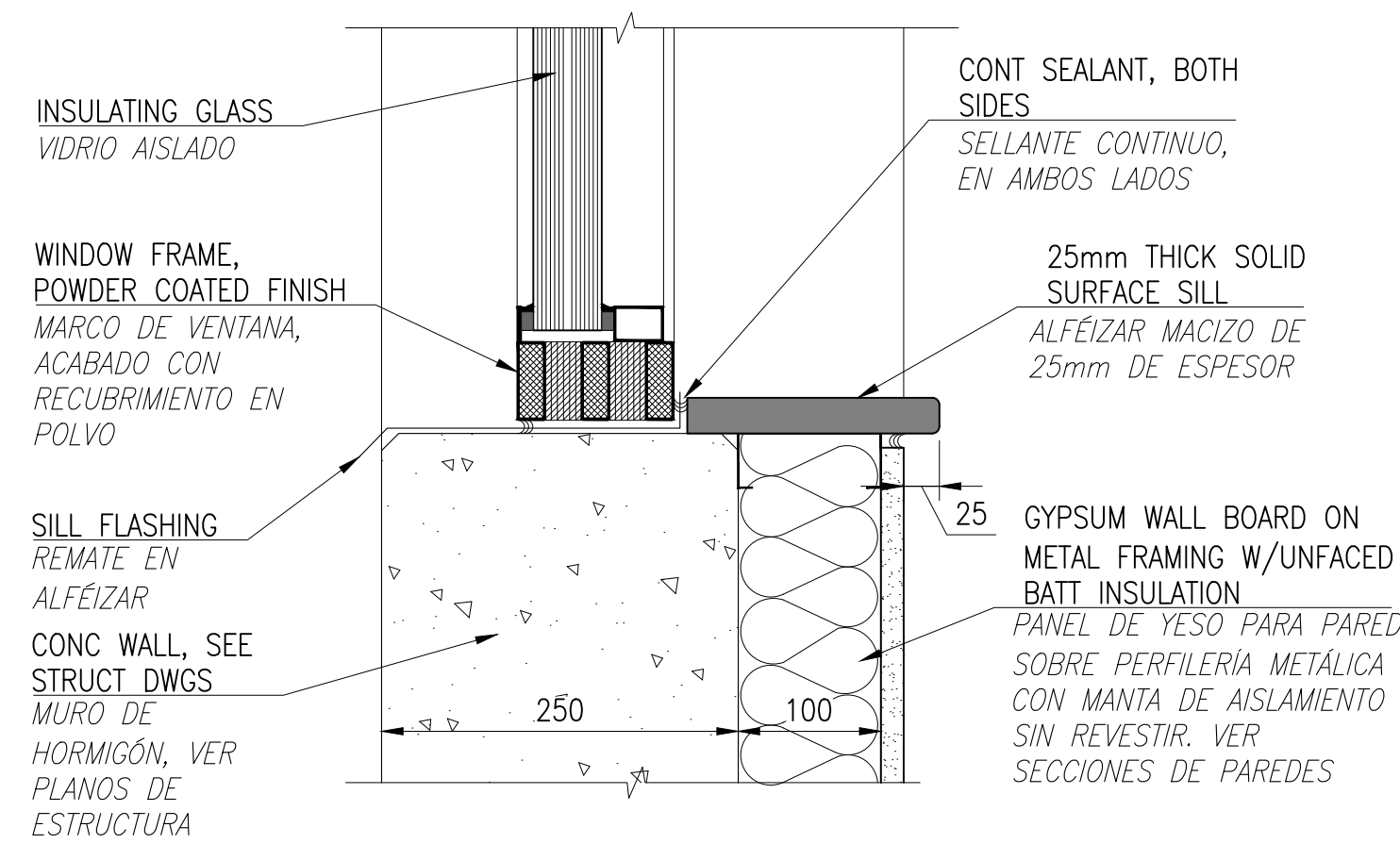
SILL DETAIL DETALLE DE ALFÉIZAR
