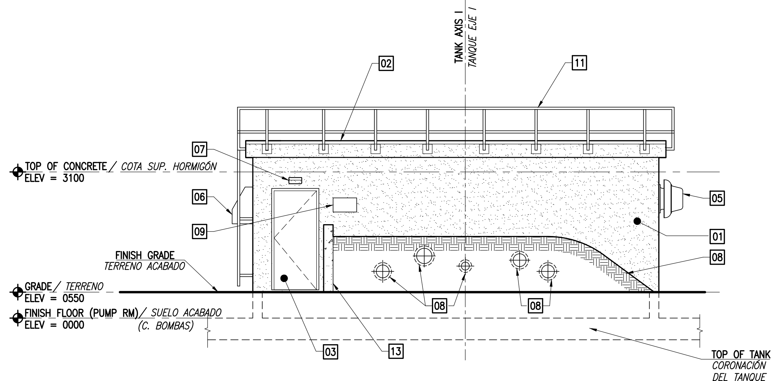
B1 ELEVATION PUMP VAULT / ALZADO CÁMARA DE BOMBAS SCALE: 1:50
