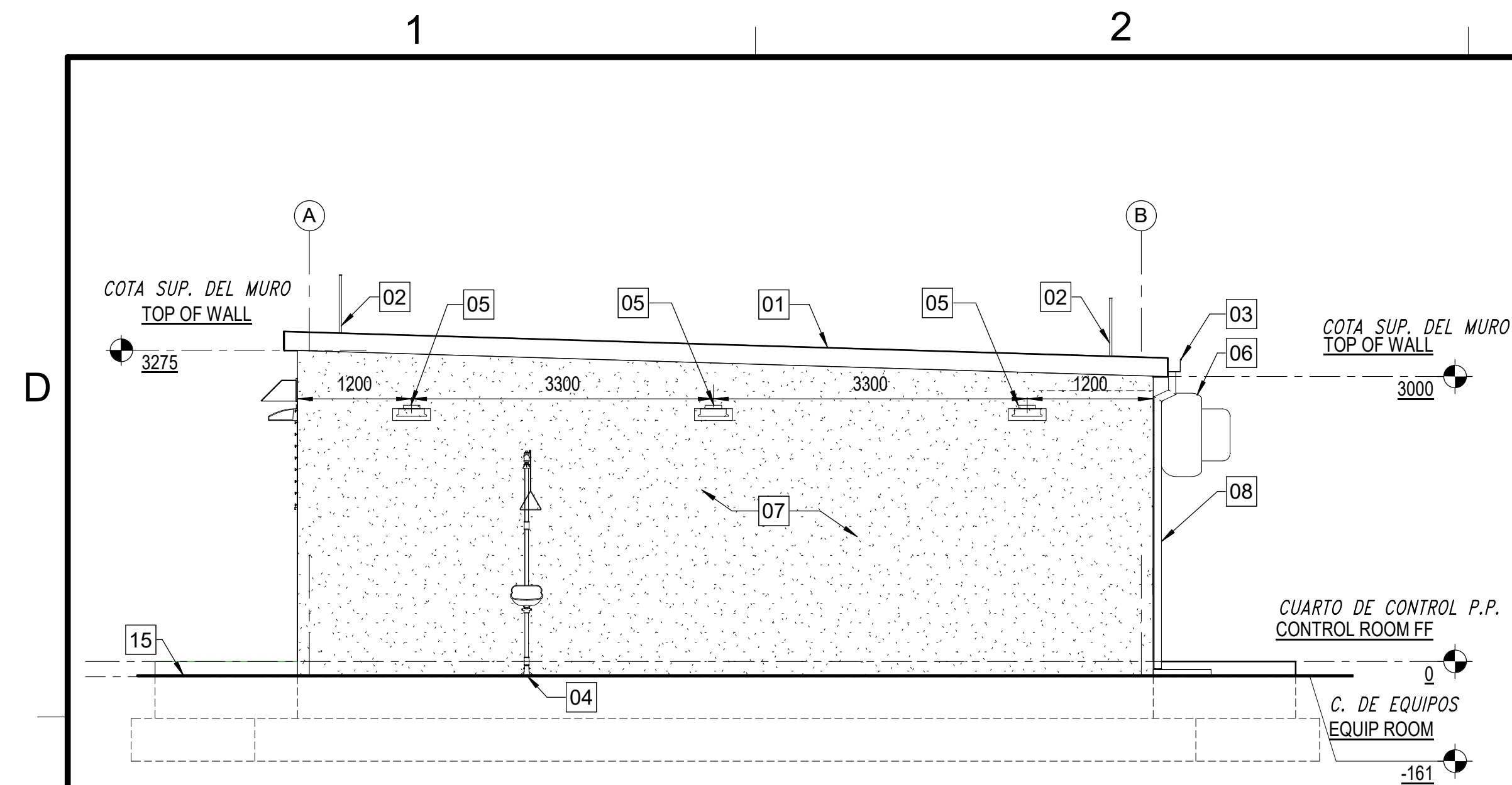
WEST ELEVATION ALZADO OESTE C1 SCALE: 1 : 50 ESCALA: 1 : 50
