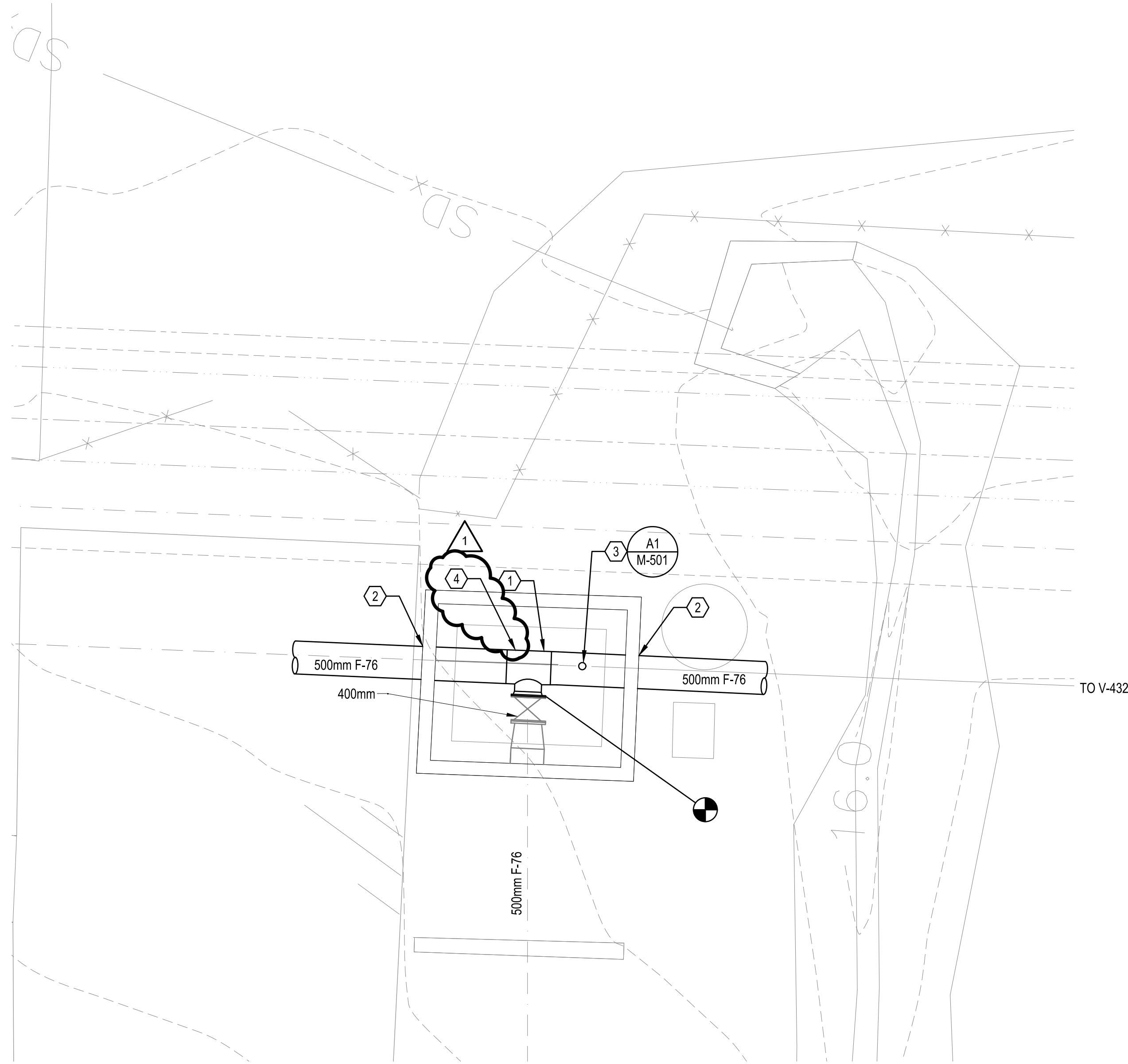
B1 PLAN - ML-1 MANHOLE PLANTA - POZO ML-1 1:50
