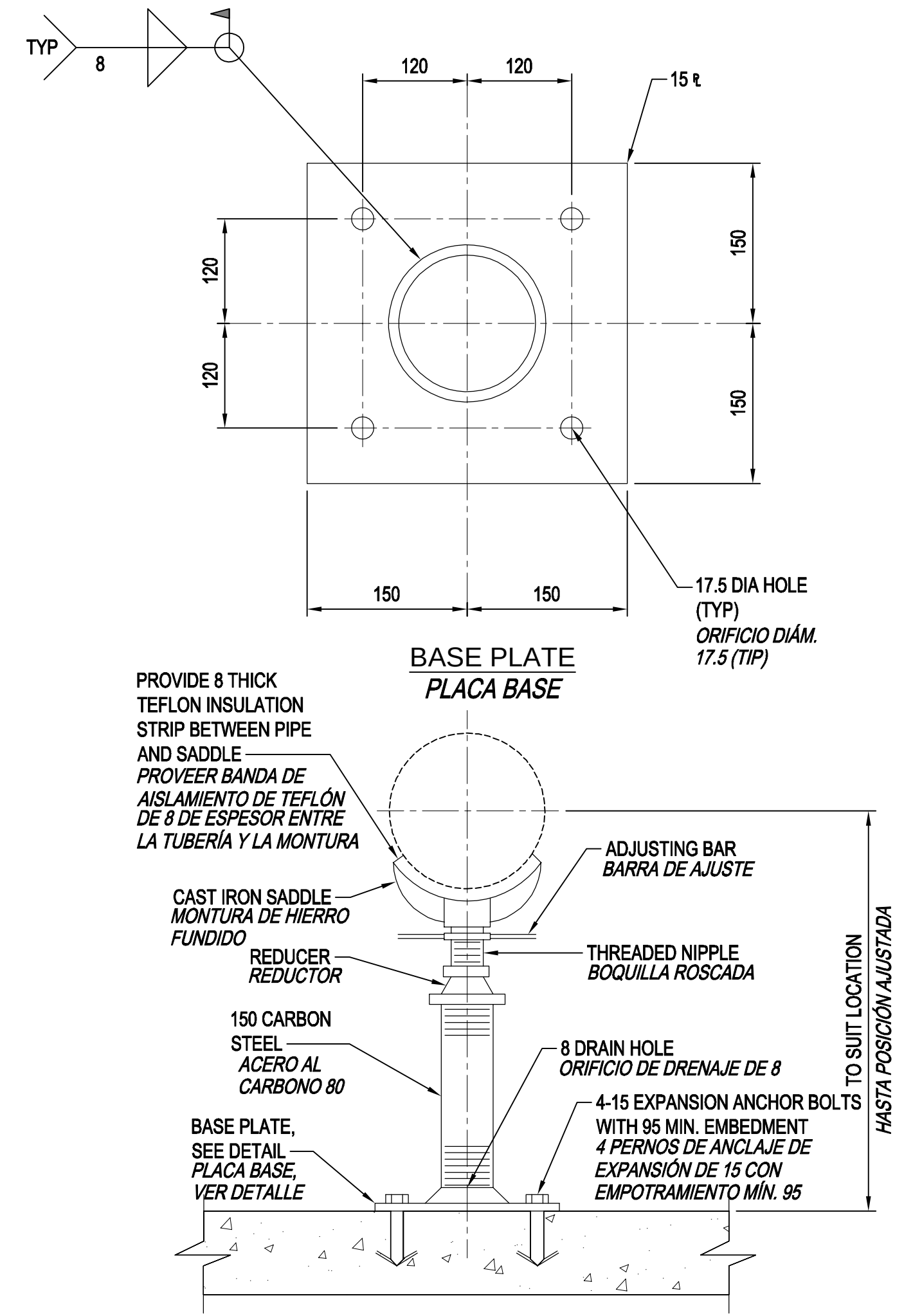
B4 ADJUSTABLE PIPE SADDLE SUPPORT DETAIL DETALLE DE SOPORTE DE MONTURA AJUSTABLE PARA TUBERÍA NTS
