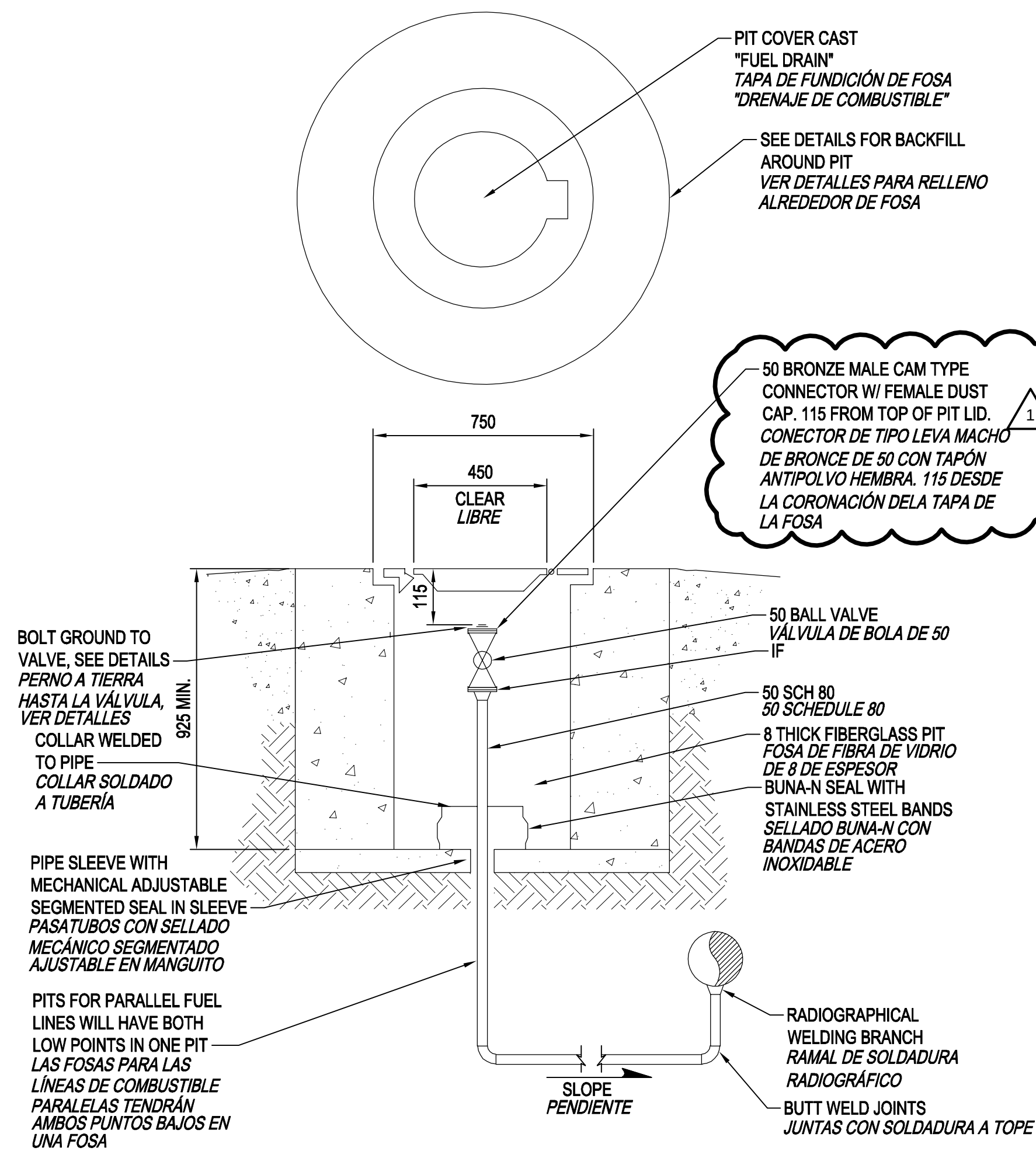
TYPICAL LOW POINT DRAIN PIT FOSA DE DRENAJE TÍPICA EN PUNTO BAJO
