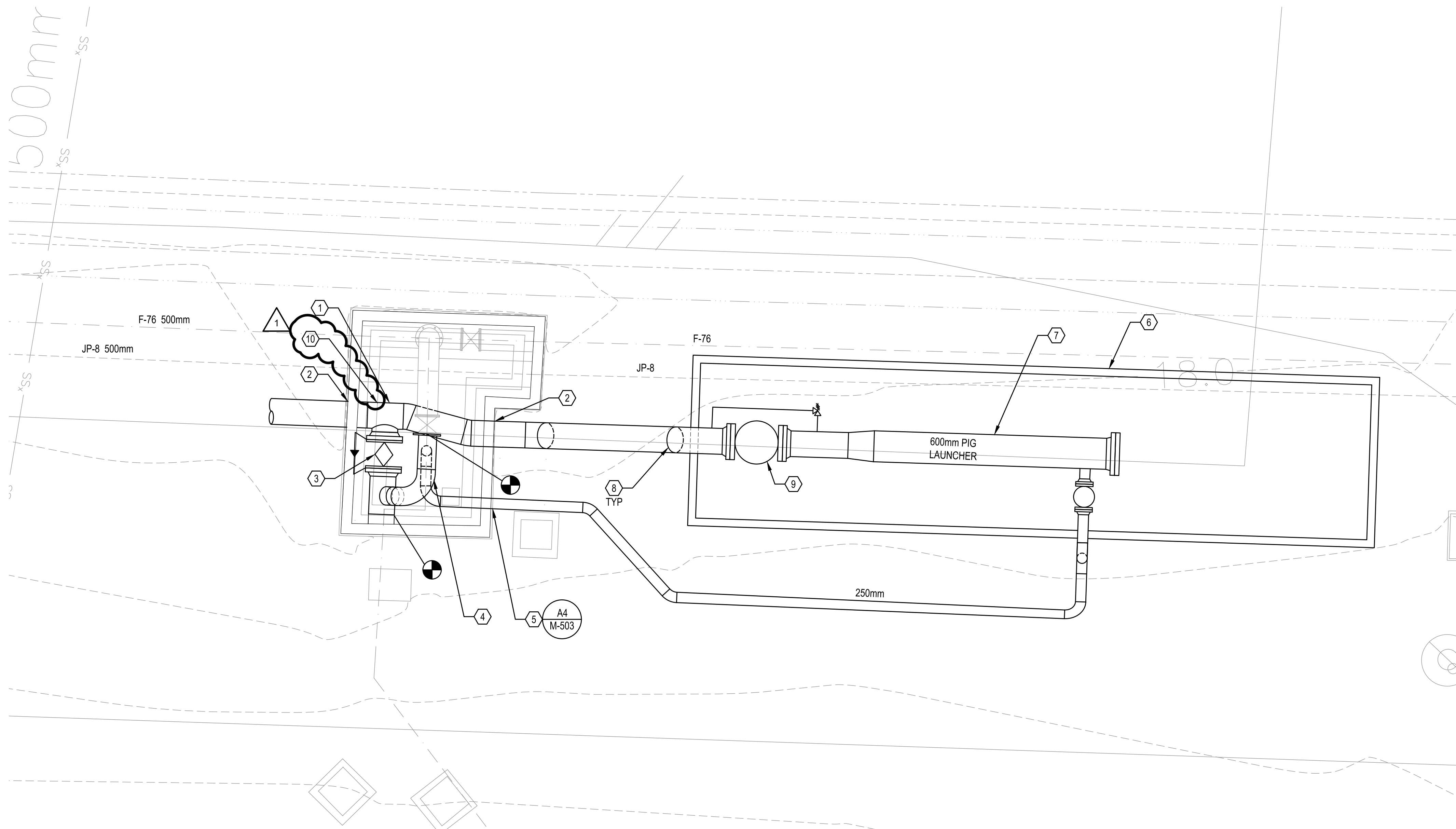
B1 PLAN - ML-2 MANHOLE PLANTA - POZO ML-2 1:50
