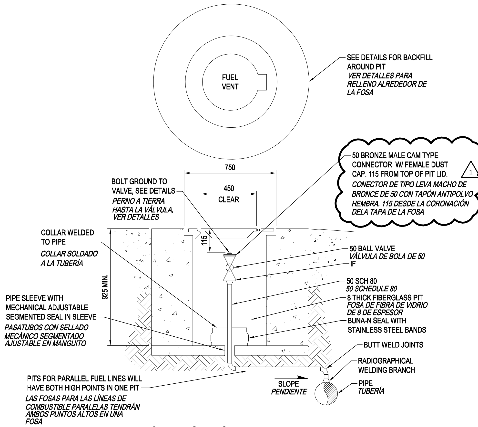
TYPICAL HIGH POINT VENT PIT FOSA DE VENTEO DE PUNTO ALTO TÍPICA
