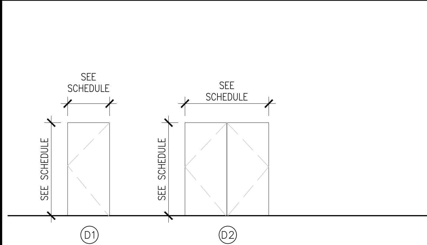
B1 DOOR TYPES SCALE: 1:50 A-606
