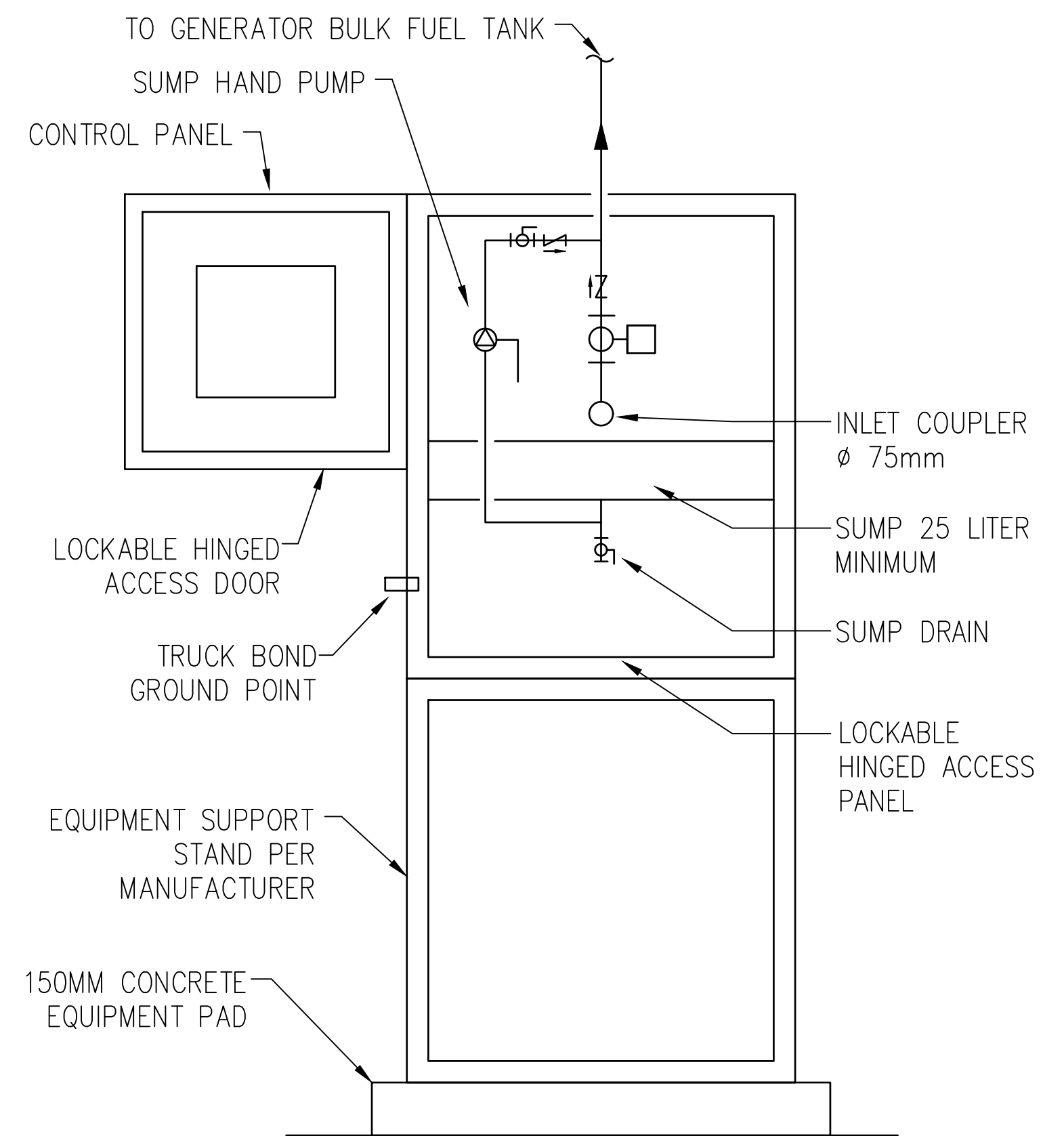
C4 AUTOMATIC FILL PORT DETAIL N.T.S.
