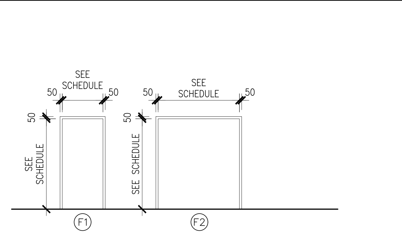
B2 DOOR TYPES SCALE: 1:50 A-606
