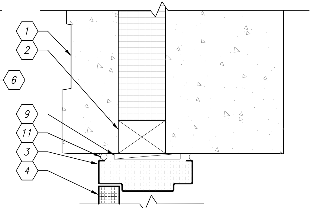
D2 EXTERIOR DOOR DETAIL - HEAD SCALE: 1:5
