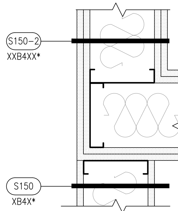
A5 2HR TO NON RATEDWALL INTERSECTION SCALE: 1:5 A-105
