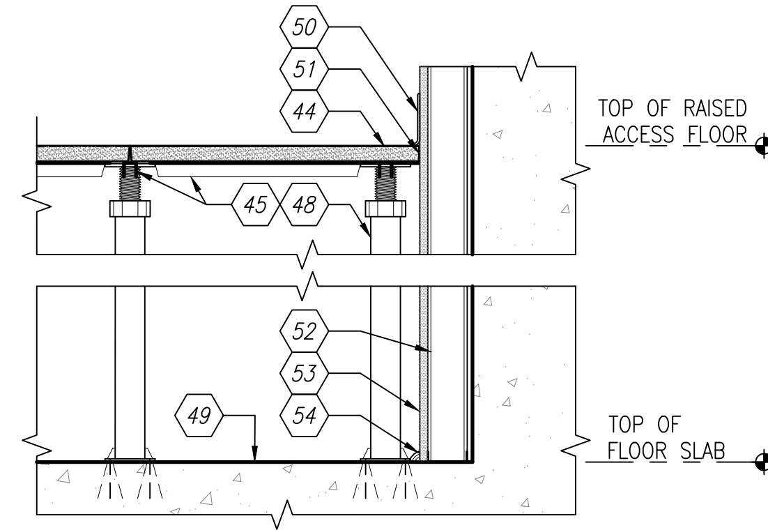
D2 ACCESS FLOOR AT CONCRETE WALL SCALE: 1:10 A-306
