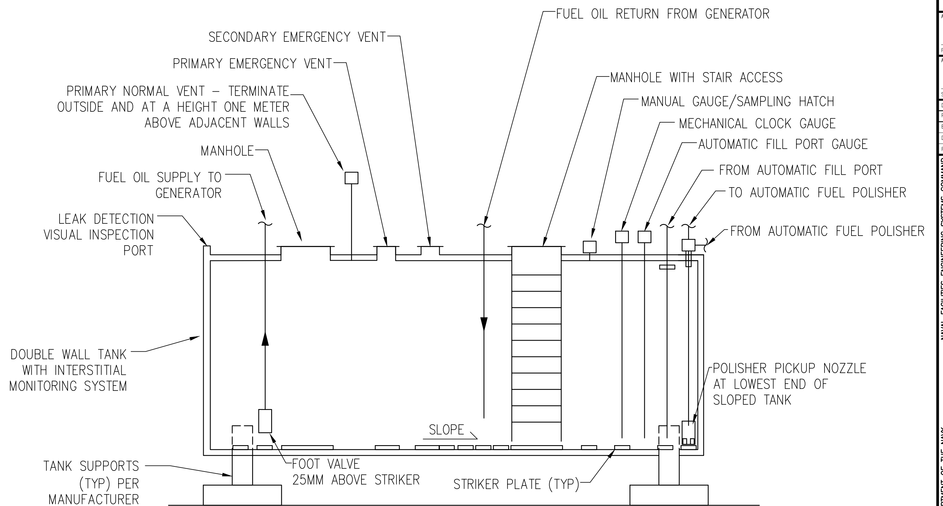
A3 GENERATOR FUEL BULK TANK DETAIL N.T.S.
