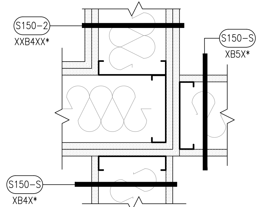
C5 2HR TO NON RATEDWALL INTERSECTION SCALE: 1:5 A-105
