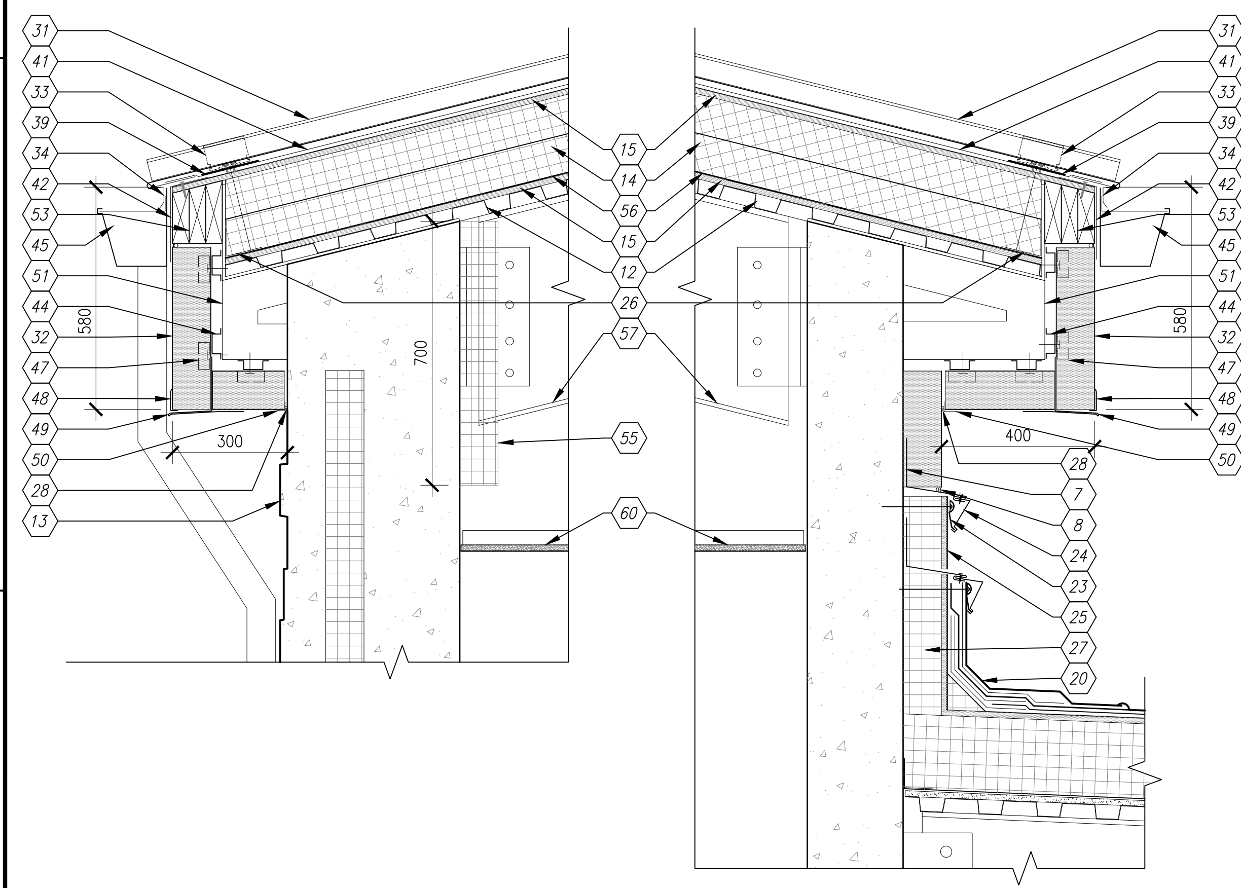
A1 HIGH ROOF EAVE DETAIL SCALE: 1:10 A-306
