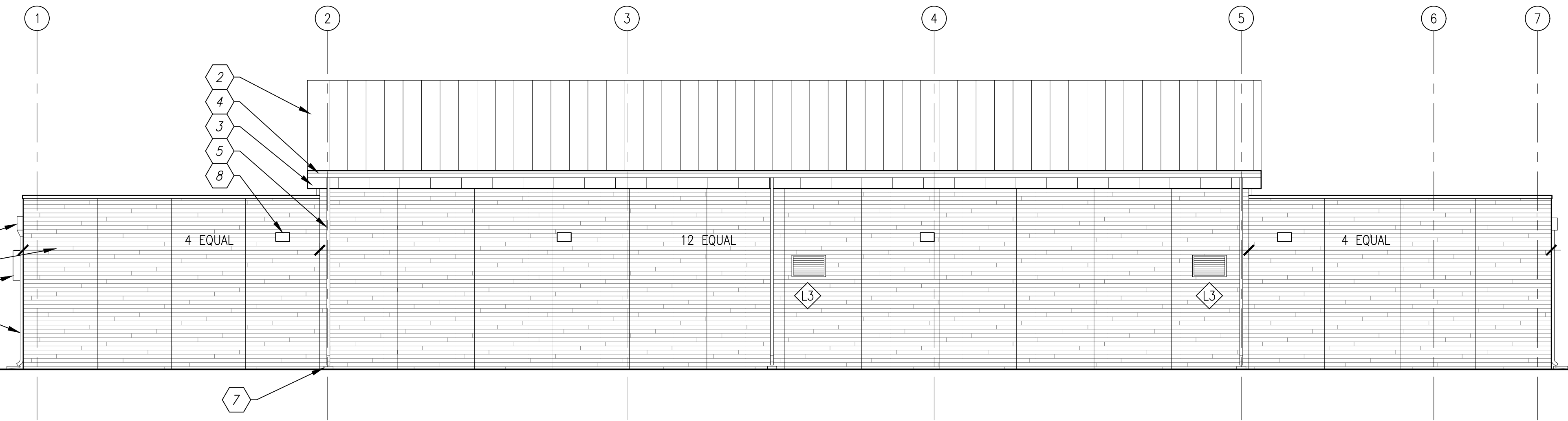
B1 NORTH ELEVATION SCALE: 1:100
