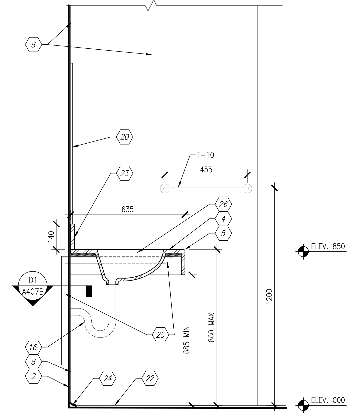
A4 SECTION AT CASEWORK - ROOM 104 SCALE: 1:10 A-406
