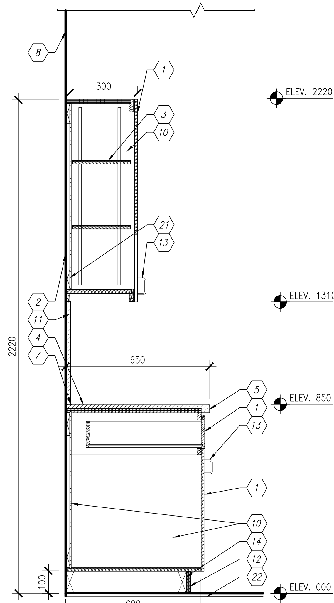
A3 SECTION AT CASEWORK - ROOM 105 SCALE: 1:10 A-406
