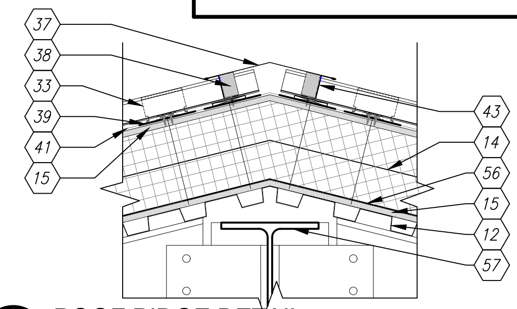
A5 ROOF RIDGE DETAIL SCALE: 1:10 A-305
