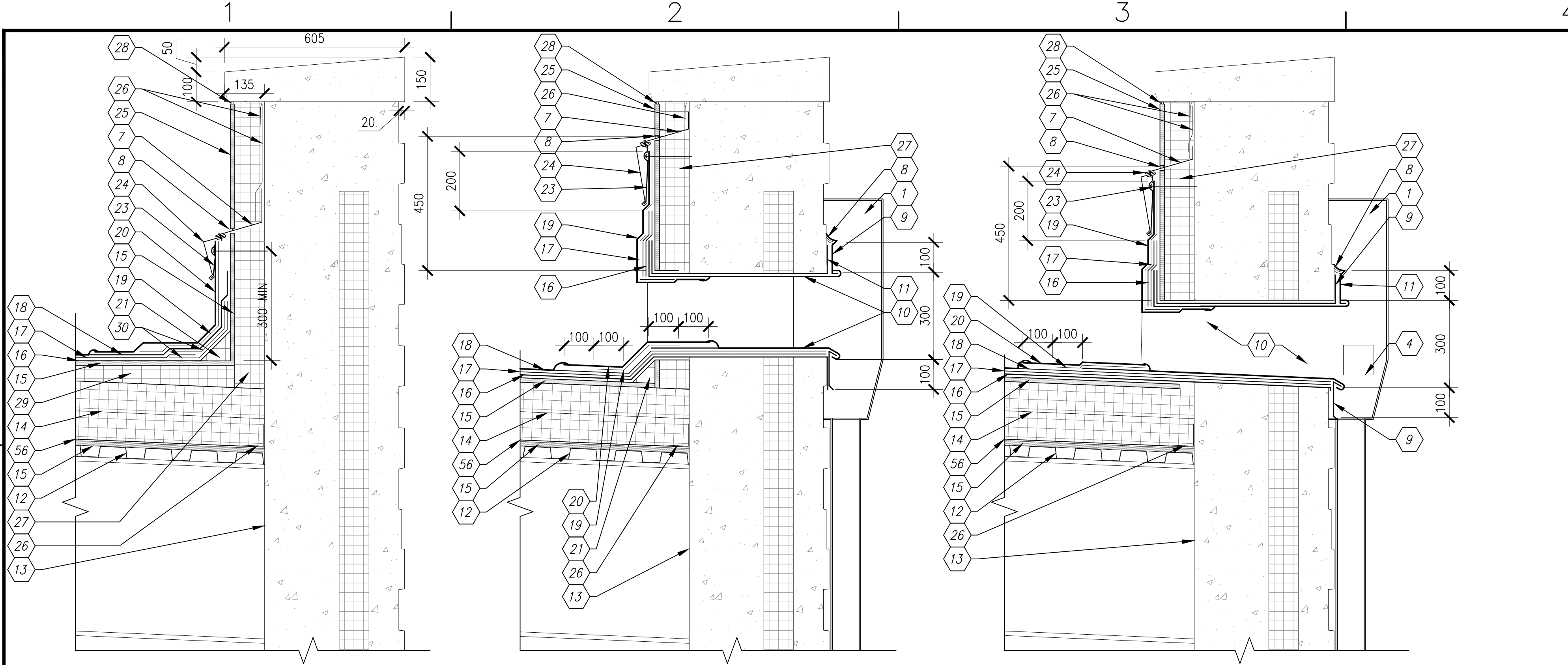
C1 PARAPET DETAIL SCALE: 1:10 A-306
