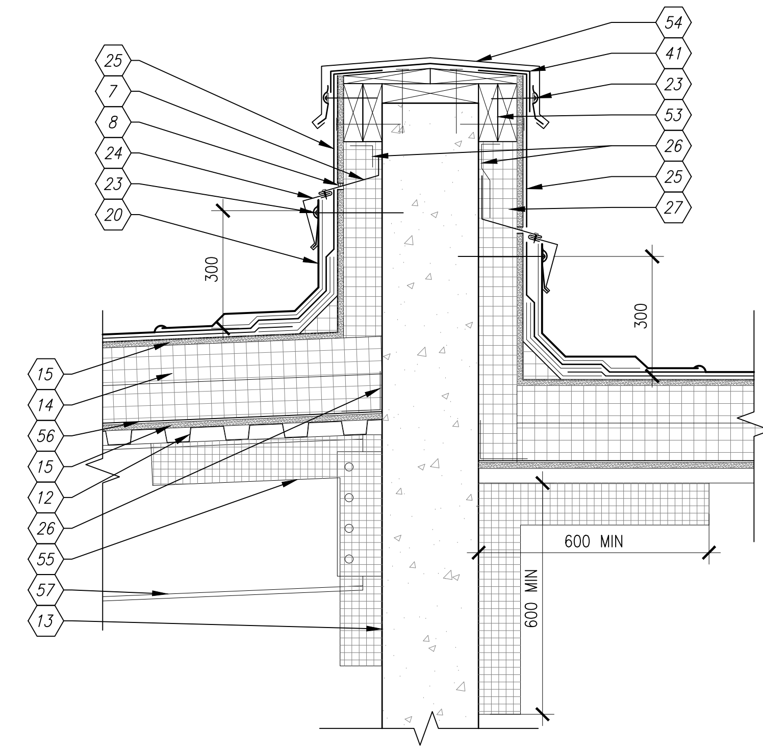
A3 ROOF CURB DETAIL SCALE: 1:10 A-107
