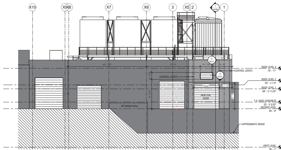
1 NORTH ELEVATION SCALE: 1/8" = 1'-0"
