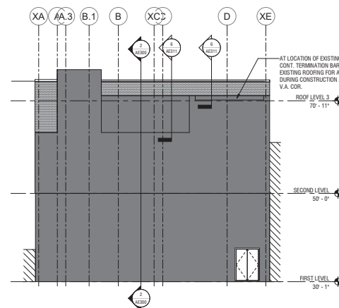
3 WEST ELEVATION SCALE: 1/8" = 1'-0"
