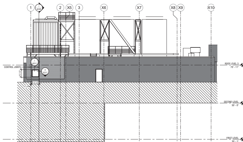
2 SOUTH ELEVATION SCALE: 1/8" = 1'-0"
