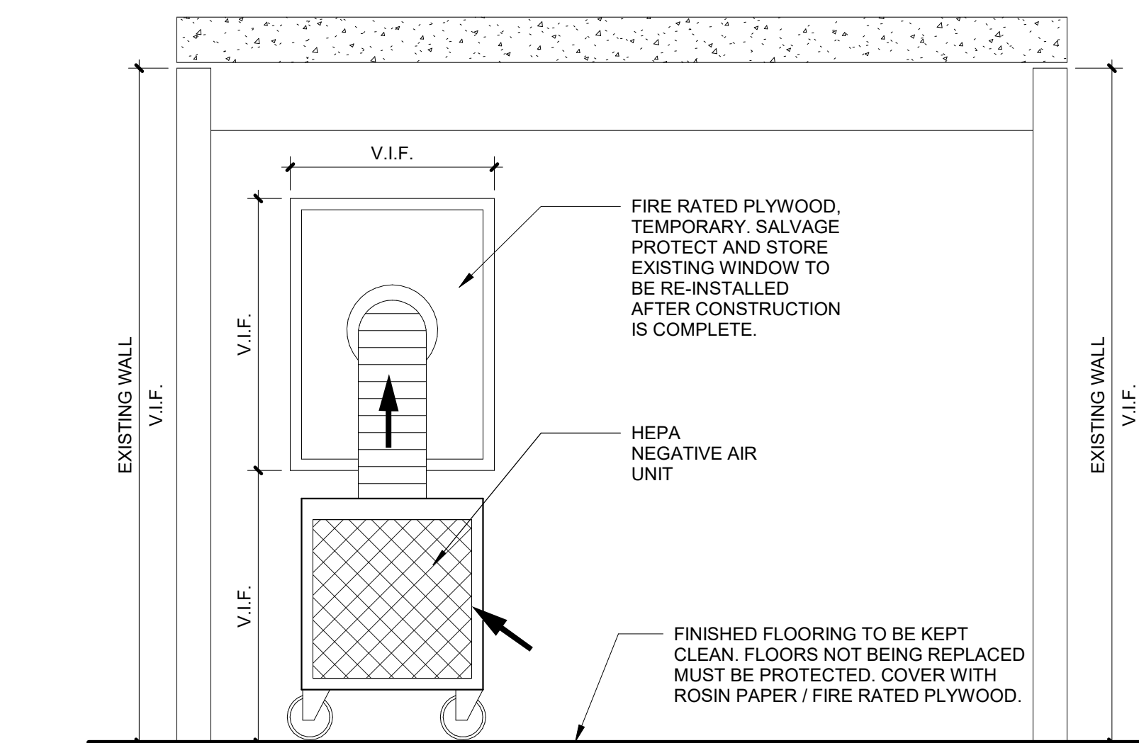
2 CROSS SECTION "A" Scale: 1/2" = 1'-0"
