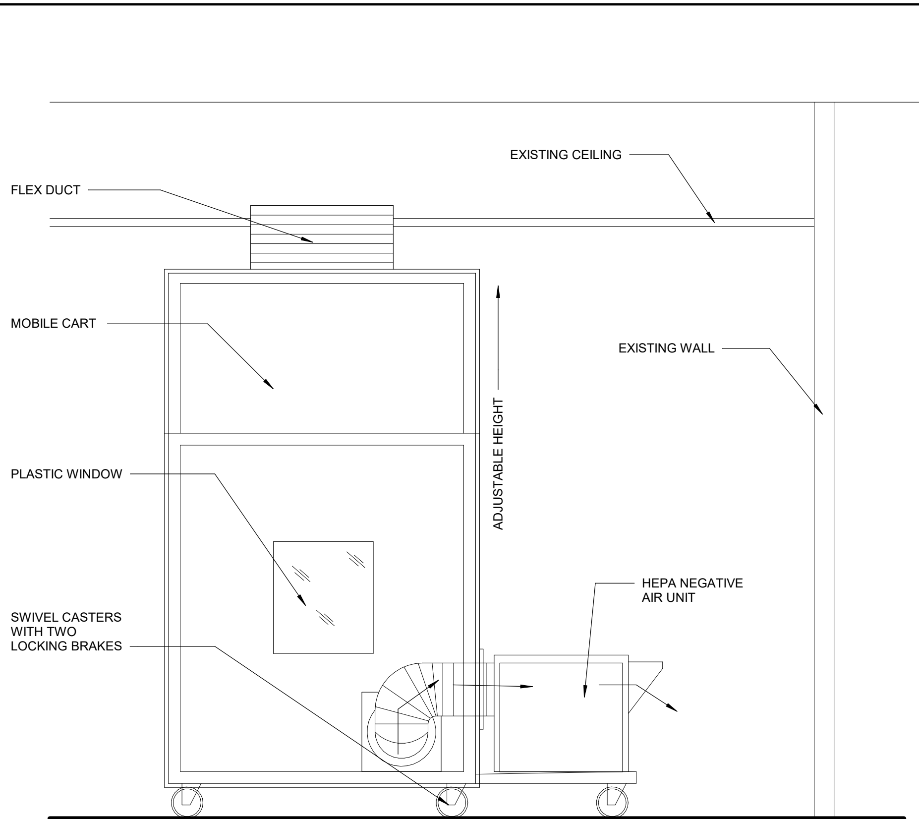
3 ICRA MOBILE CONTAINMENT CART Scale: 1/2" = 1'-0"
