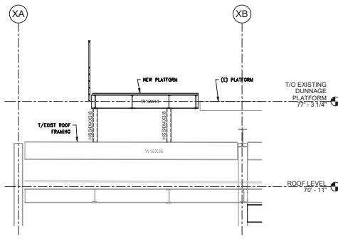
3 SECTION SCALE: 3/8" = 1'-0"
