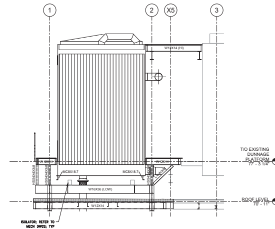
3 SECTION SCALE: 1/4" = 1'-0"
