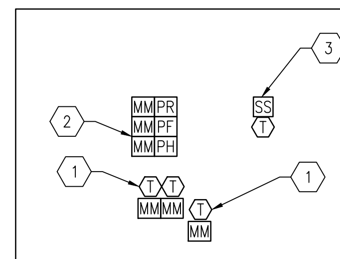
A3 FIRE ALARM PUMP ROOM 113 SCALE: 1:100
