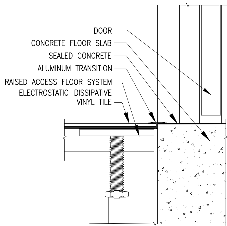
D4 RAF TRANSITION SCALE: 1:5 IN601
