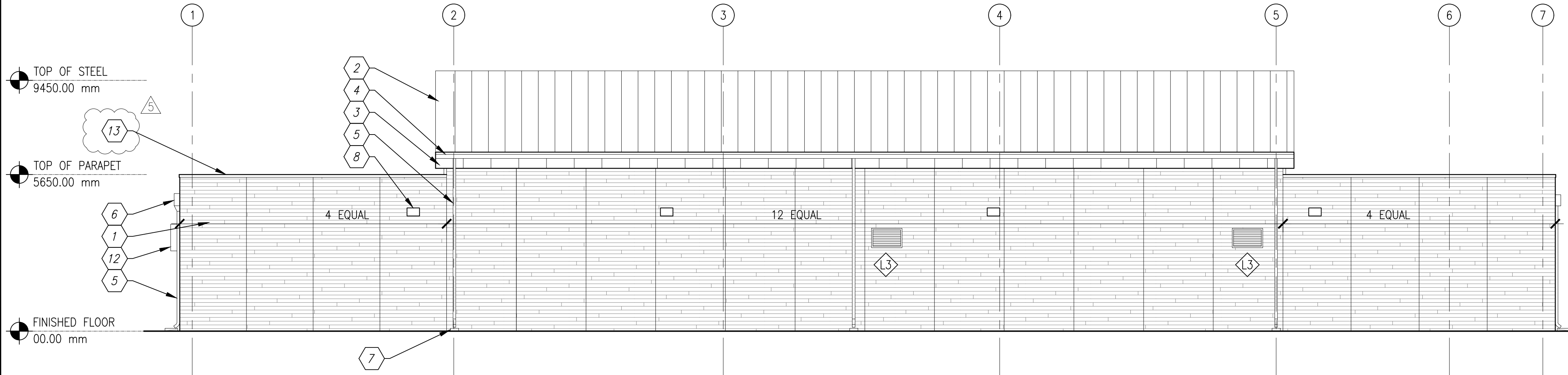
B1 NORTH ELEVATION SCALE: 1:100
