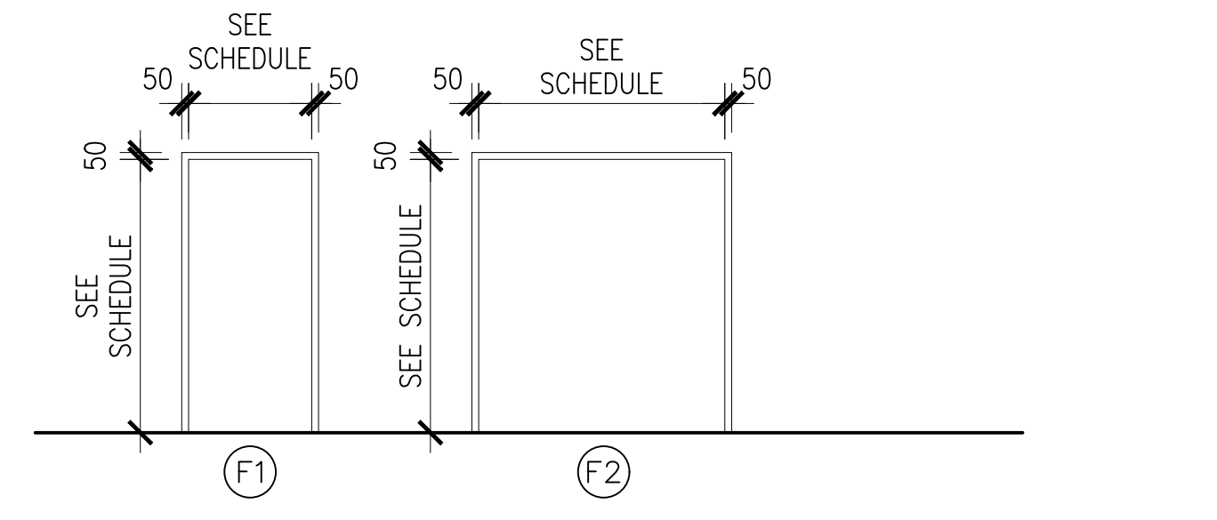
B2 DOOR TYPES SCALE: 1:50 A-606
