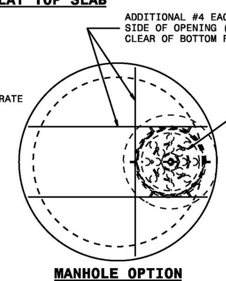
MANHOLE OPTION
