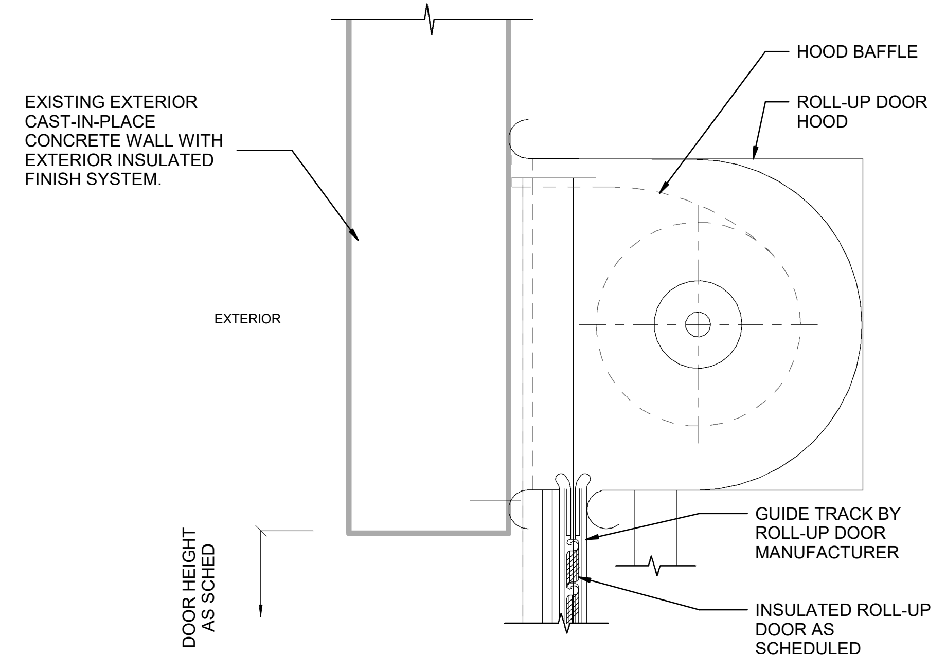
E7 OVERHEAD COILING DOOR HEAD DETAIL 1:5
