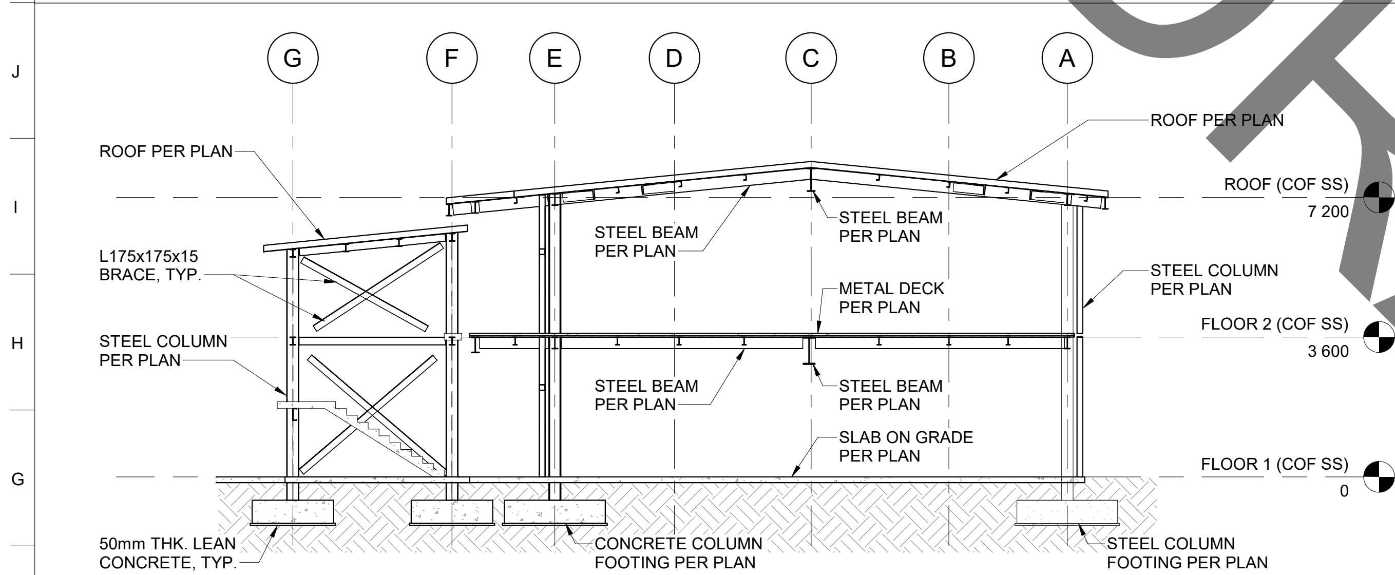
F1 COF SS - BUILDING SECTIONS (CLIN 0004) SCALE 1 : 100
