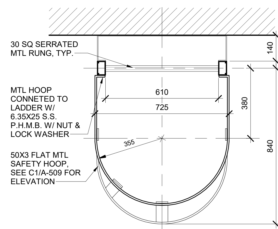
A8 CAGE PLAN 1 : 10
