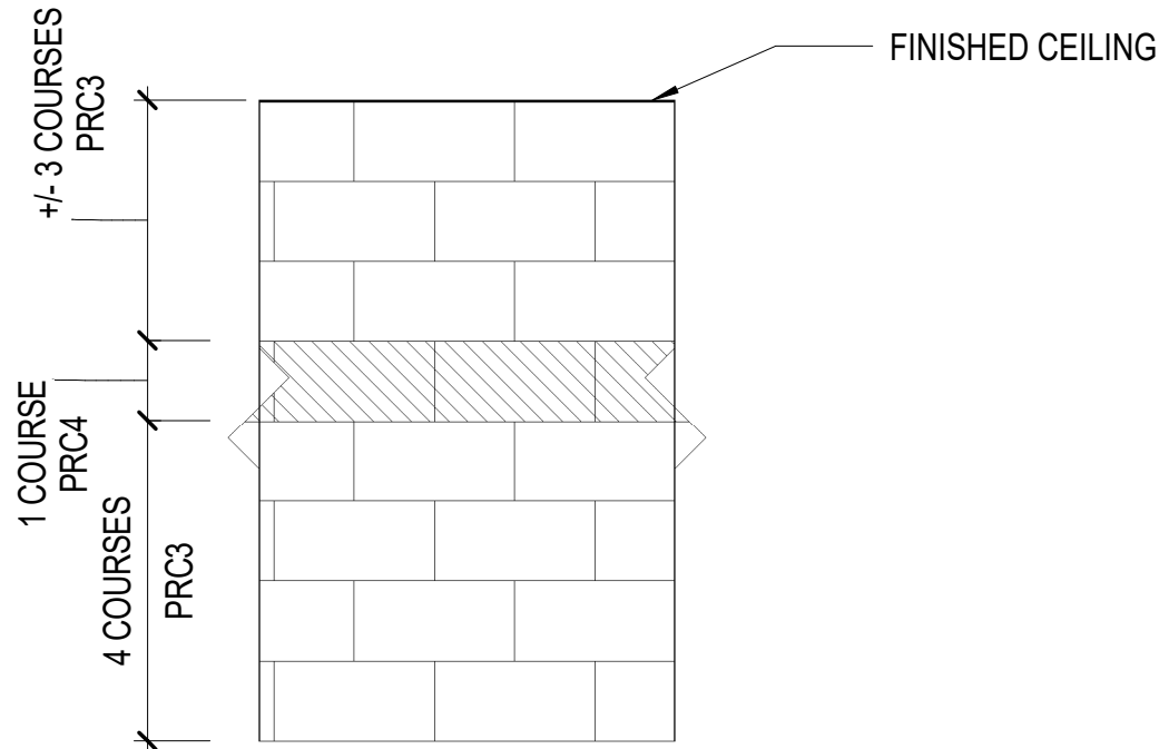
D1 WALL TILE ELEVATION TYP 3/8" = 1'-0"
