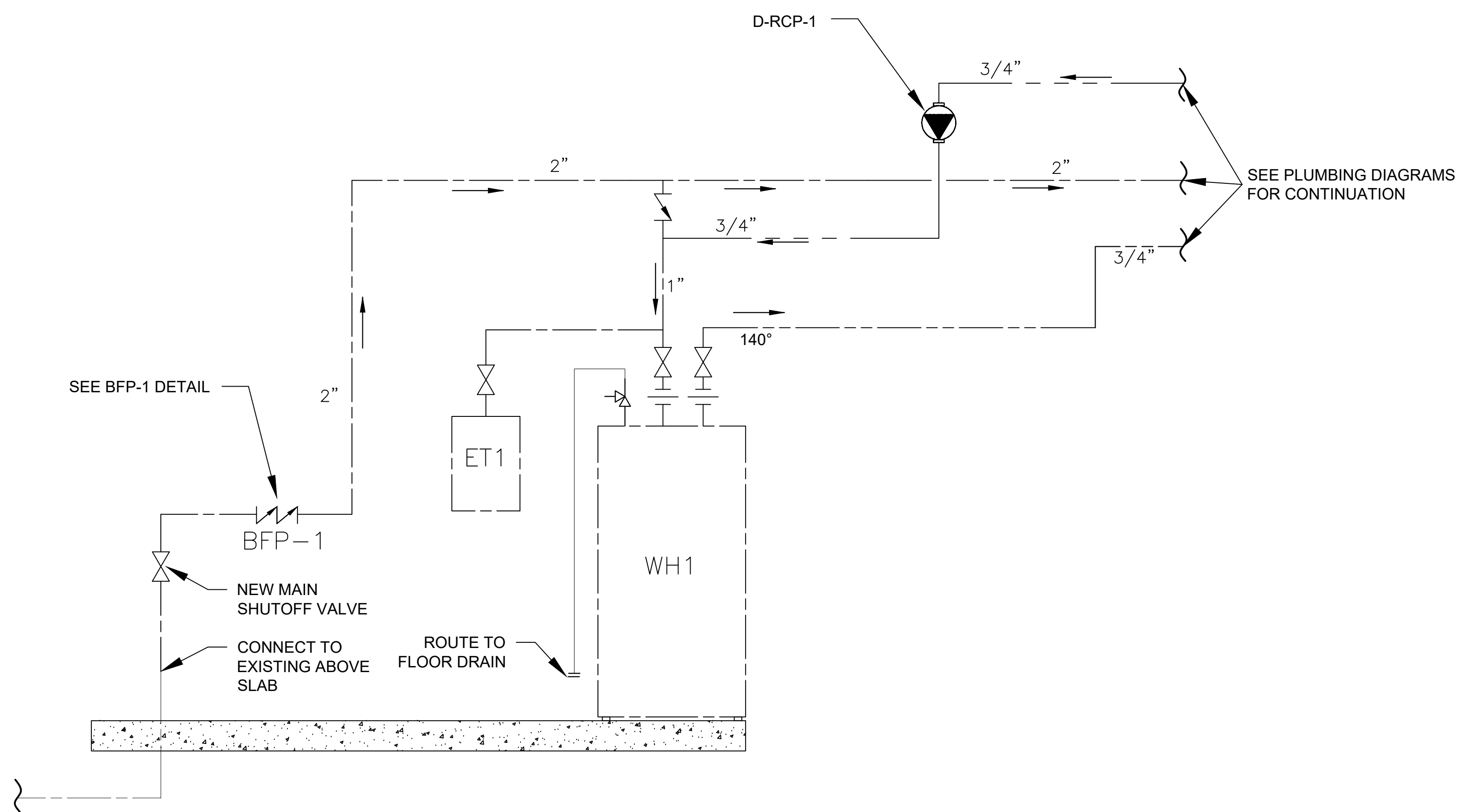
D1 WH-1 DETAIL NTS
