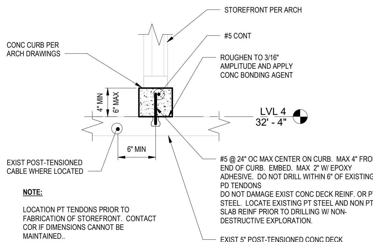
E1 CONC CURB DETAIL 1" = 1'-0"
