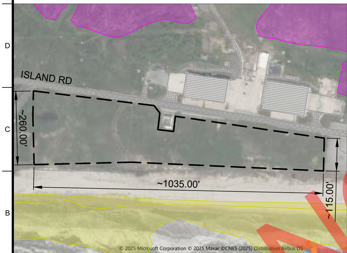
A1 LAYDOWN AREA 4 1" = 200'-0"
