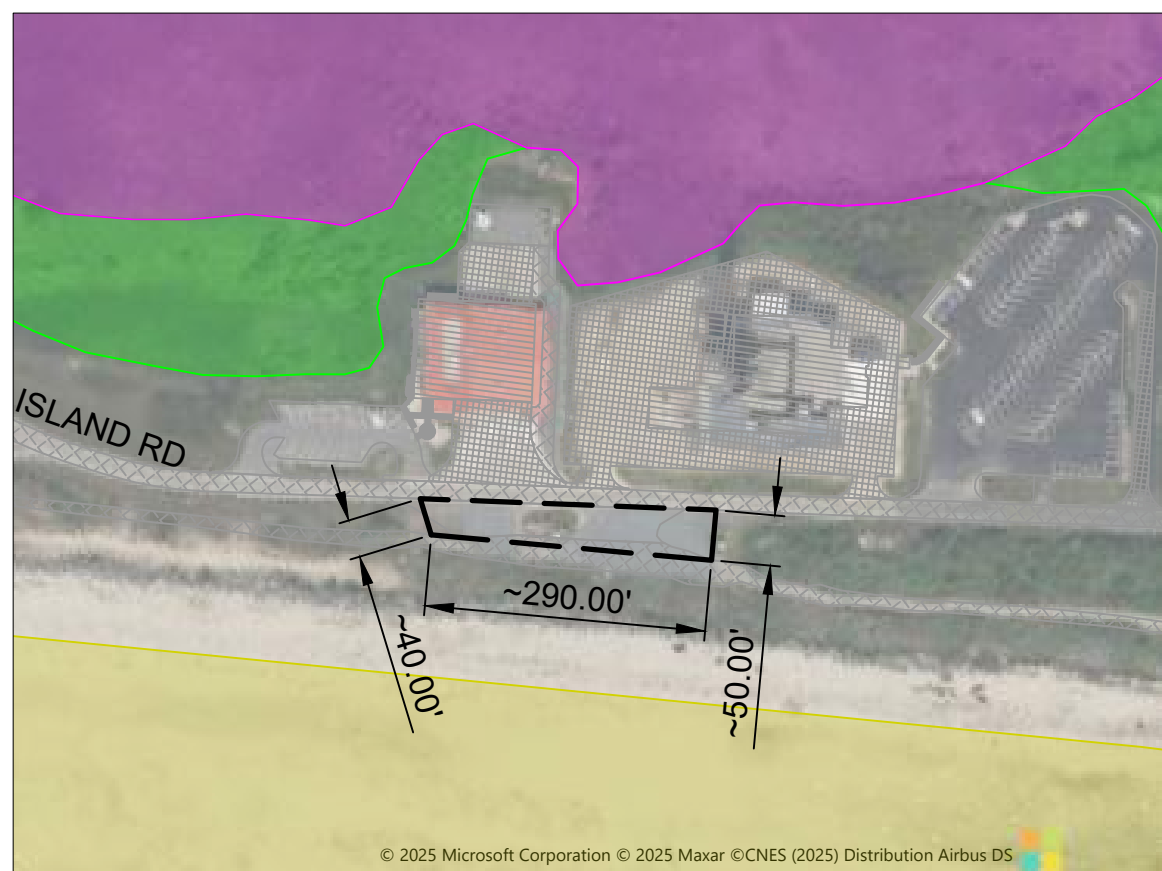
A13 LAYDOWN AREA 6 1" = 200'-0"
