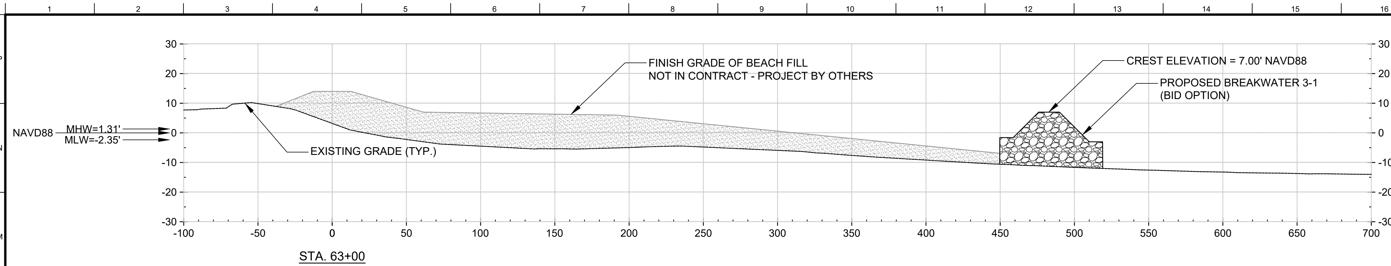
BREAKWATER 3-1 STA 63+00
